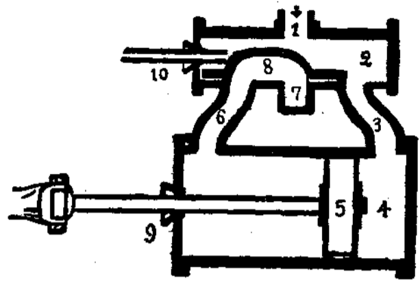
汽缸剖面圖
