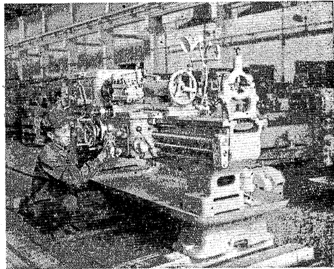
沈陽市目前有16個機械工廠正為越南、越南、朝鮮生產170多架(件)機械設備。這是沈陽第一機床廠為越南生產的一A六二車床。(新華社記者于 攝)
