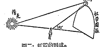
圖二：虹霓的形成。
