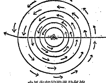
台風內部的漩渦狀氣流
