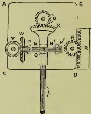
FIG. 3.—Sectional plan.
