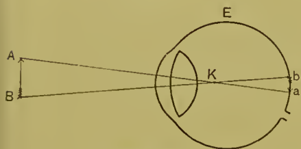
Visual angle.
