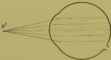
Position of anterior focus.
