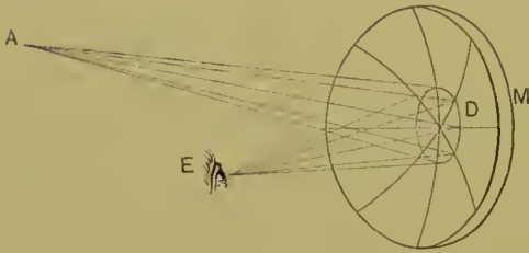
Real image.
