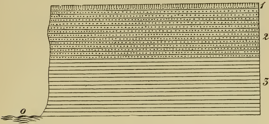
Fig. 3. Perfil de la Barranca de los Lobos á medio kilómetro al sur de la Bajada Martínez de Hoz. 0, nivel del Atlántico; 1, tierra vegetal; 2, piso ensenadense; 3, piso chapalmalense.
