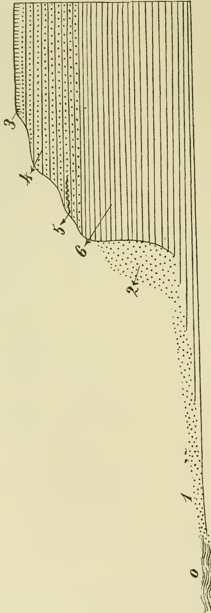
Fig. 9. Perfil de la barranca á unos 8 km. al norte de la Bajada Martinez de Hoz. O, nivel del mar; 1 Arena de la playa; 2, depósito de arena acumulada por el viento contra la base de la barranca; 3, tierra vegetal; 4, ensenadense; 5, banco calcáreo de la transgresión interensenadense; 6, chapalmalense.
