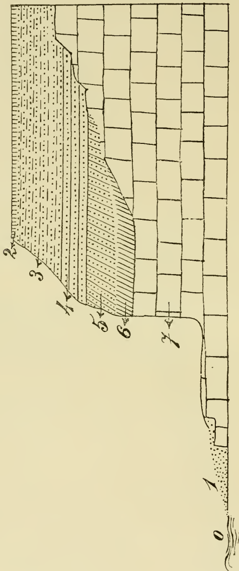
Fig. 11. Perfil del barranco del extremo oeste de la cantera de Punta Porvenir. 0, nivel del Atlántico; 1, arena de la playa; 2, tierra vegetal; 3, bonaerense; 4, ensenadense cuspidal; 5, depósitos eolomarinos contemporáneos del intersensadense; 6, banco marino de la transgresión intersensadense; 7, cuareta silúrica.
