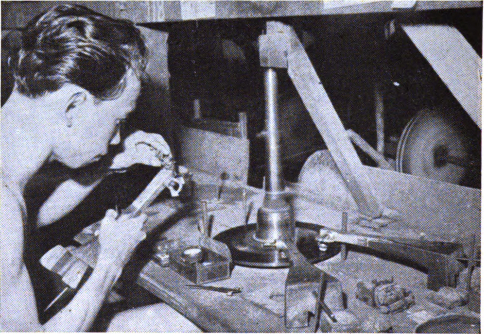
Gurindam dijalankan dengan tenaga listrik. Seorang pekerdja sedang melihat hasil penggosokannya.
