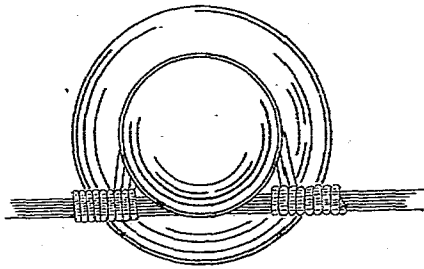
磁頭紮綫平面圖
