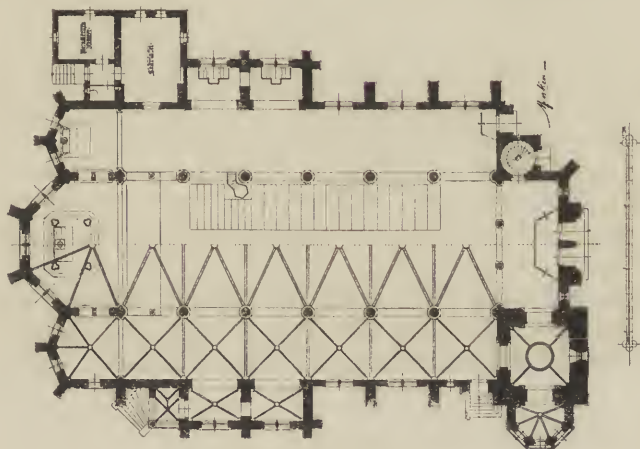
Abbildung 1 (Grundriss).
