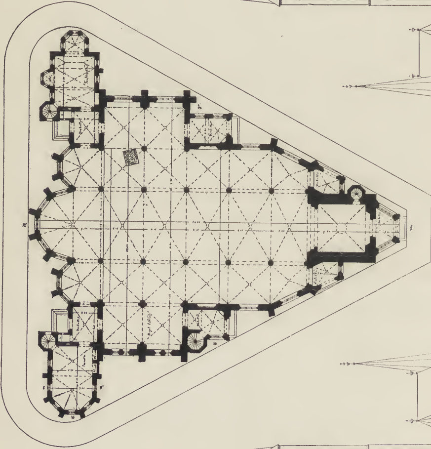
Grundriss.
