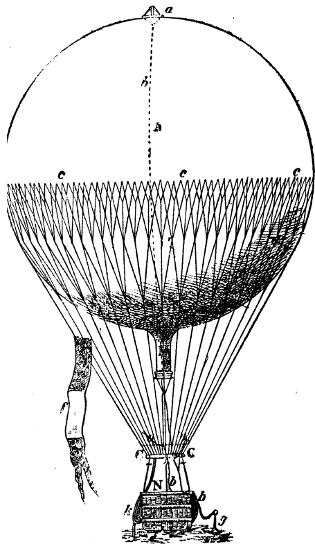
Фиг. 1. А—баллонъ; М—аппендиксъ, или ручка; СС—кольцо; N—корзина; а—клапанъ; б—клапанная веревка; с—сѣтка; к—гайдропъ; h—якорная веревка; г—якорь; f—флагъ.
