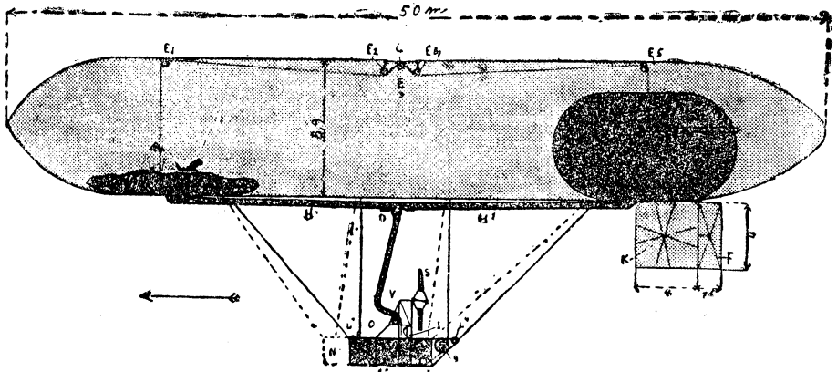
Фиг. 5. V^1 —передній, V^2 —задній баллонетъ; H^1 , H^2 —рукава для подачи воздуха въ баллонетъ отъ вентиля D . V —вентиляторъ для пополненія баллонетовъ. E^1 , E^2 , E^3 , E^4 , E^5 —блоки, черезъ которые перекинута веревка, соединяющая баллонеты; если пусты оба, то, такъ какъ роликъ E^3 соединенъ со спускающимъ газъ вентиляемъ G , то этотъ послѣдній открывается. St —стабилизаторъ. K —киль. F —руль поворота. S —винтъ. N —гондола. N^1 —положеніе гондолы во время полета. L^1 до L^4 —блоки для канатъ въ, поддерживающихъ гондолу. R —резервуаръ для бензина.
