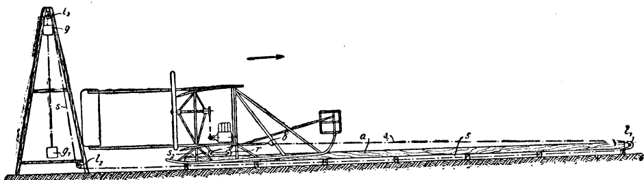
Фиг. 25. Стартъ Райта. а—брусъ для разлета съ роликомъ l_1 , черезъ кот. проведенъ канатъ s , для приведенія въ движеніе аэроплана по бусу. Канатъ привязывается къ аэроплану за крюкъ b , и какъ только веревка, удерживающая грузъ g , опускается и самый грузъ падаетъ въ положеніе g_1 , веревка s влечетъ аэропланъ; l_2 , l_3 —направляющіе блочки на башнѣ старта; г —ролики на кареткѣ старта.
