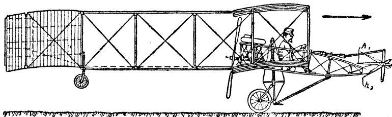
Фиг. 26. Разлетъ аэроплана Фарманъ-Буазентъ. Заднія колеса поднимаются, разлетъ совершается на переднихъ. Послѣ того какъ руль глубины переложенъ будетъ изъ положенія h_1 въ положеніе h_2 , начинается подъемъ.
