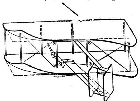
Фиг. 24. Поддержив. поверхности и руль поворота въ аэропланѣ Райта, когда онъ описываетъ кривую влево (перспективный видъ).
