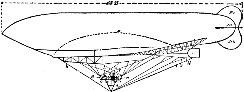
фиг. 7. К—киль. F—стабилизаторъ и руль поворотовъ. Н—руль высоты. St 1 до St 3 —стабилизир. плоскости. а—баллонеты. N—гондола съ моторомъ M. Z—зубчатая передача къ винту T. W—охлажд. аппаратъ. R—резервуаръ для бензина.
