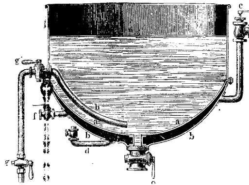
3. Дефекаціонный котель.
