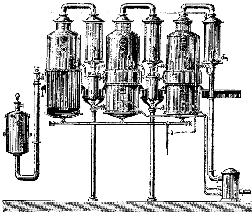
7. Выпаривательный аппарат Роберта.
