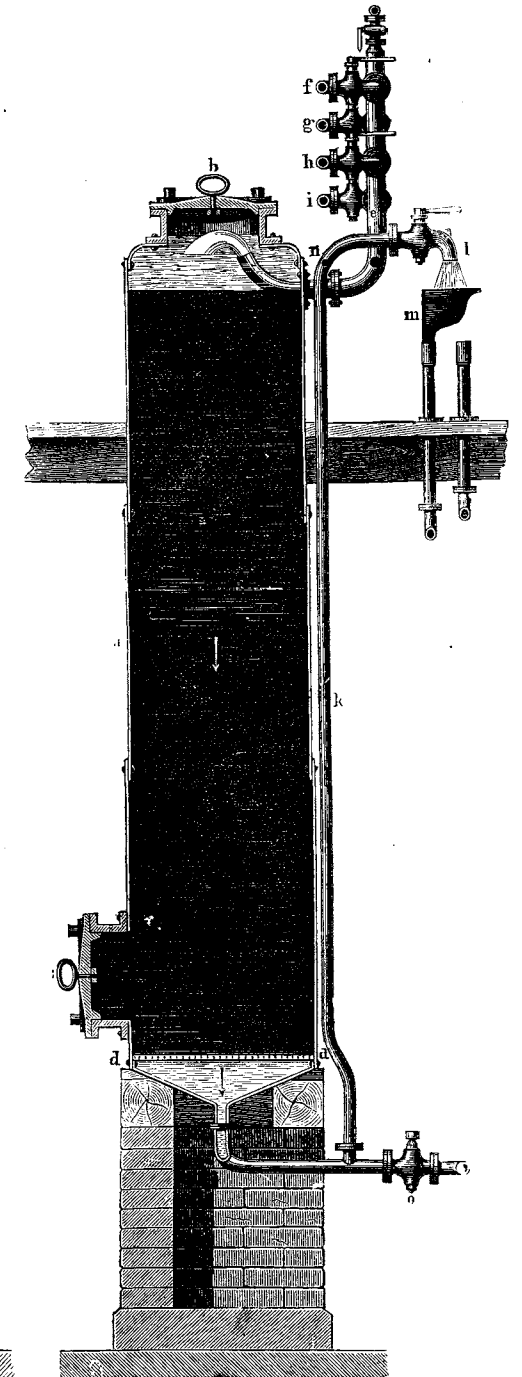
6. Колонна изъ костяного угля.
