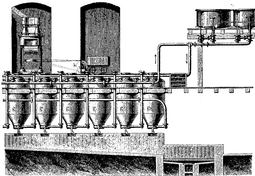
2. Диффузионная батарея.
