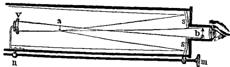
Рис. 3. Рефлекторъ Грегори.
