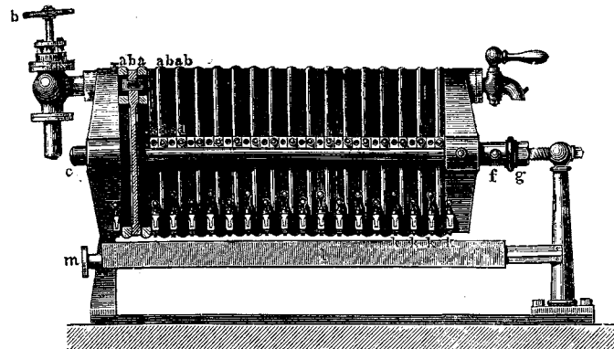
5. Филтрпрессъ.
