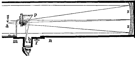
Рис. 1. Рефлекторъ Ньютона.
