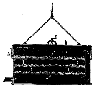
6. Разрѣзь очистительнаго ящика.
