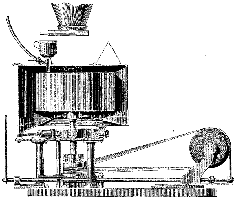
9. Центрофуга.
