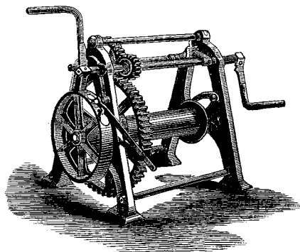
Лебедка.
