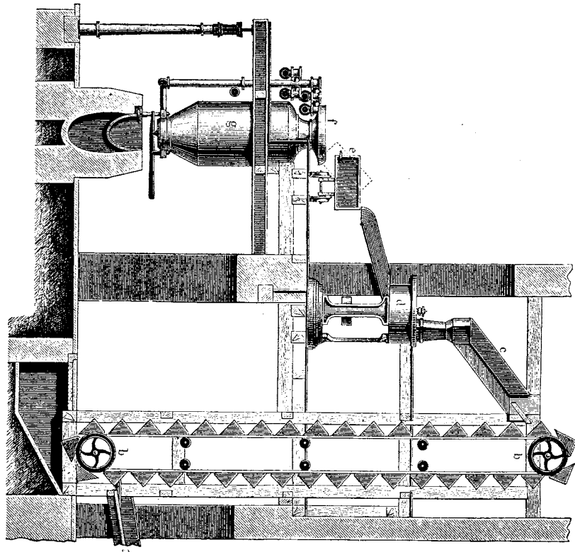
1. Диффузионная батарея (боковой видъ)
