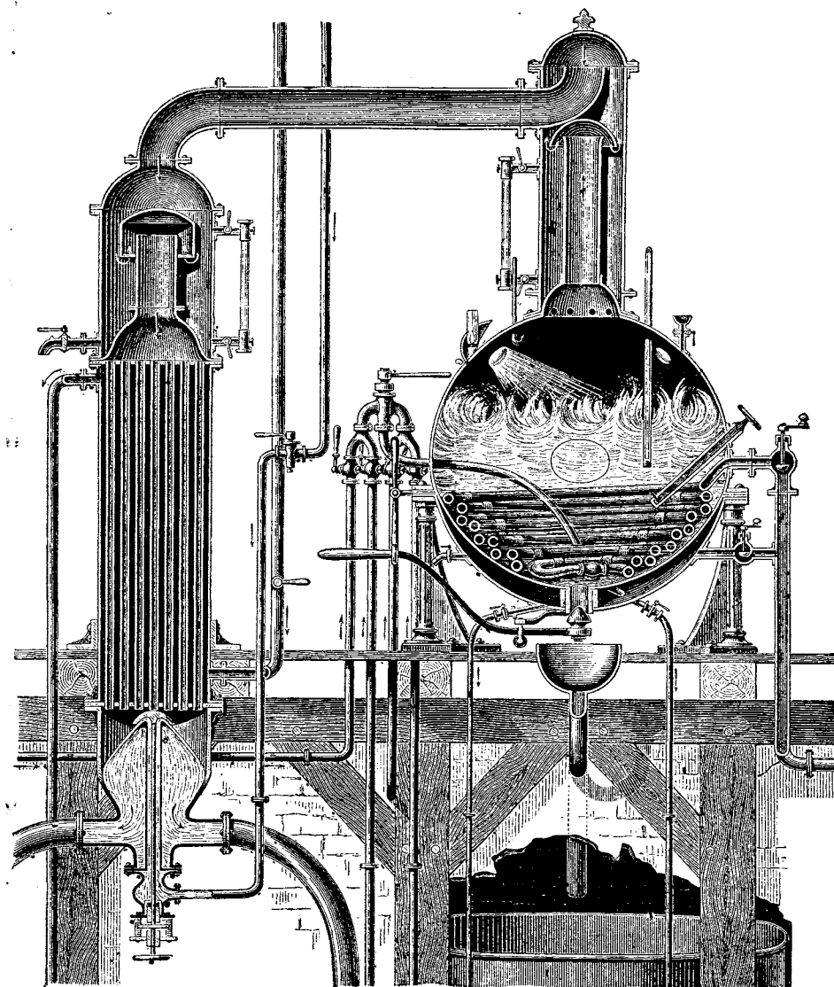
8. Вакуум-аппаратъ.
