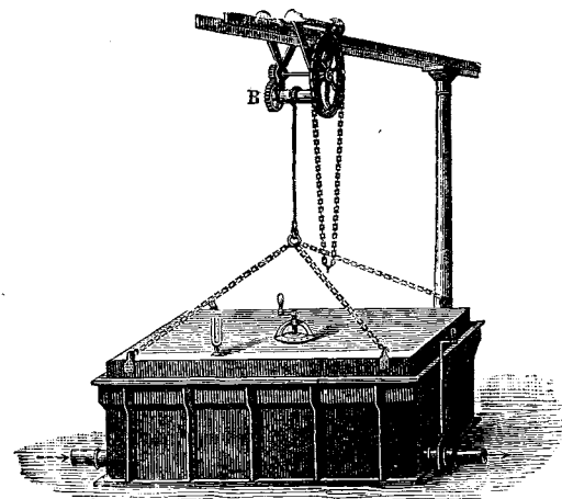
5. Очистительный ящикъ.
