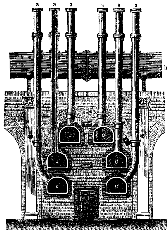
1. Реторты.
