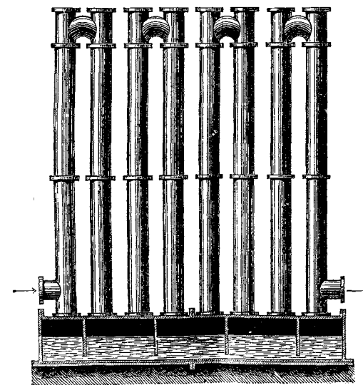
3. Холодильники.
