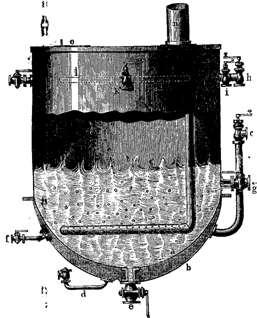
4. Сатураціонный котель.
