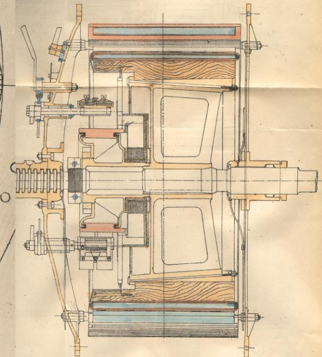
Coupe par l'axe longitudinal.
