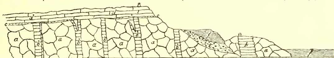
Fig. 1. — a) roccia basaltica alterata; b) dicchi; c) conglomerato; d) calcare senoniano; e) conglomerato vulcanico; f) arenarea calcarea.
