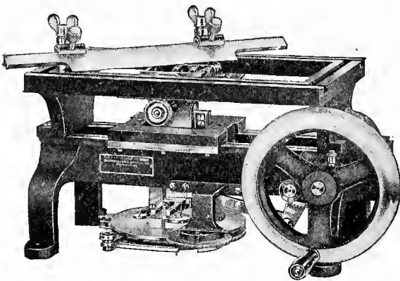
FIG. 107.—Minot precision microtome (Bausch & Lomb).
