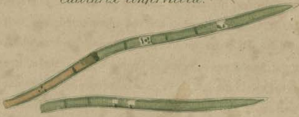
Calothrix confervicola.
