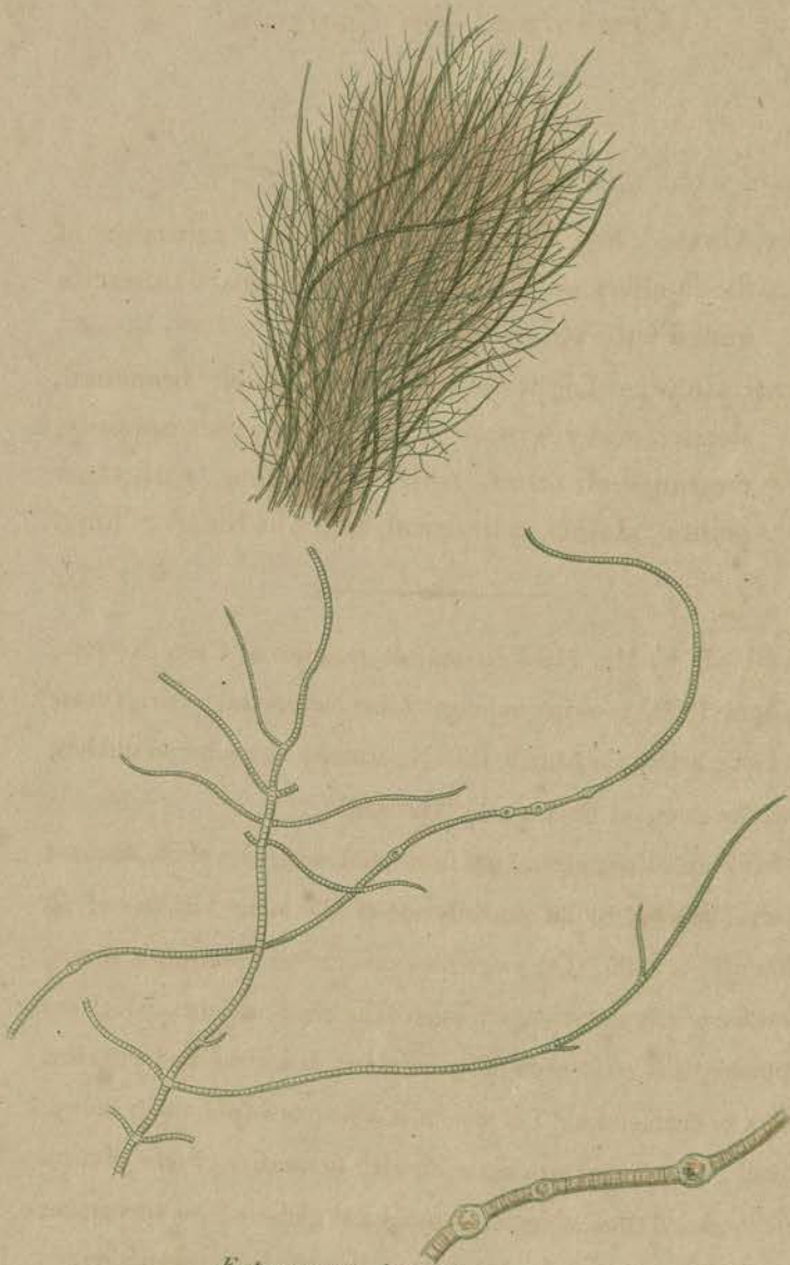
Ectocarpus brachiata?
