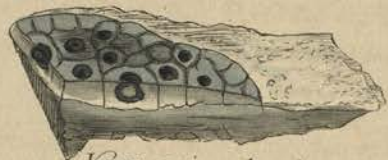
Verrucaria plumbea.
