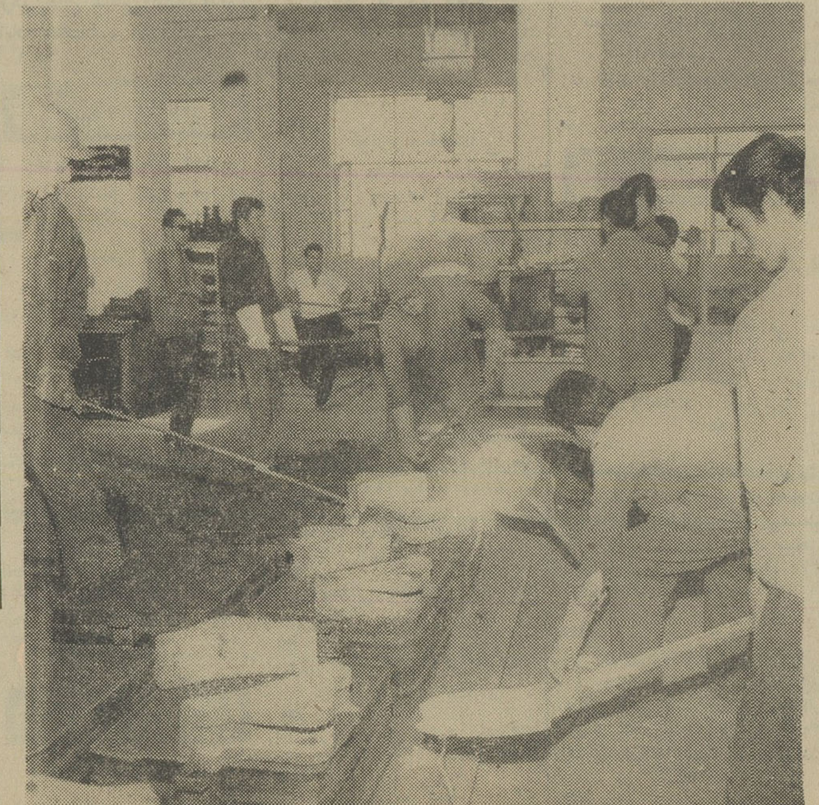
از کوره ذوب آهن، راه آهن مانند کوره مخصوص ساخت ابزار یدکی میریزند بزرگ آهن و فولاد مذاب را در قالبهای
