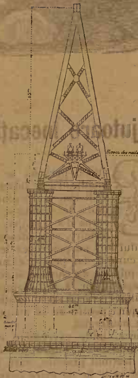
Plan vertical a unei pile la podul de peste Mâneca.
