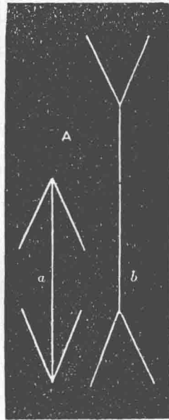
第十八圖 Müller-Lyer 的錯覺
