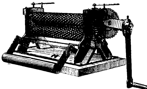
Вальцы Сист. Perfectionnè.
