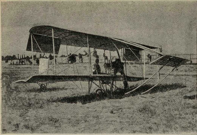
Аэропланъ А. С. Кудашева.
