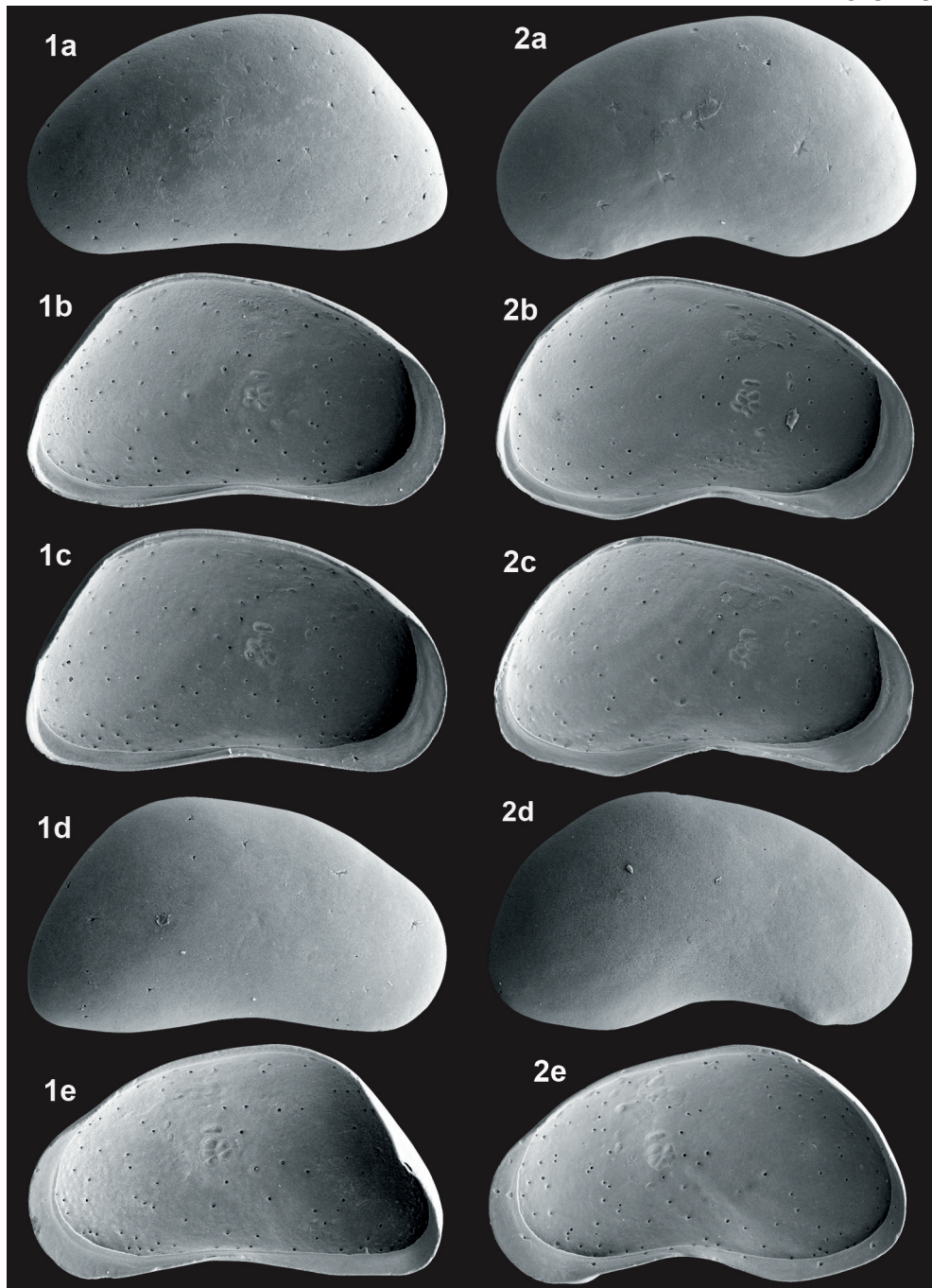
Fabaeformiscandona levanderi (HIRSCHMANN, 1912) – Großstorkwitz (18) mWKz Weibchen: 1a - LVa (L 1,14), 1b - LVi (L 1,10), 1c - LVp (L 1,05), 1d - RVa (L 1,07), 1e - RVi (L 1,07), Männchen: 2a - LVa (L 1,17), 2b - LVi (L 1,16), 2c - LVp (L 1,17), 2d - RVa (L 1,24), 2e - RVi (L 1,21).
