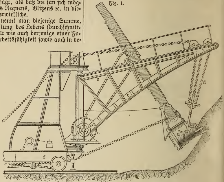
Erntator von Ruston, Proctor u. Komp.
