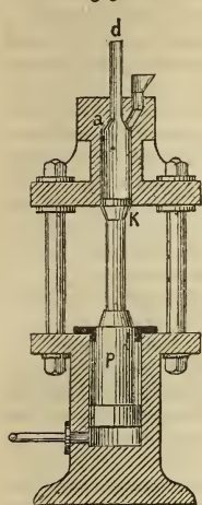
Drahtpresse.
