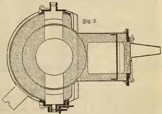
Rigar's Kupolofen. Querschnitt.
