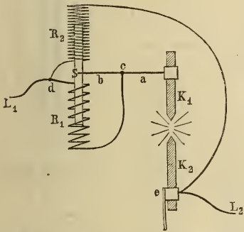
Schematische Darstellung der elektrischen Differentiallampe von Hefner-Alteneck
