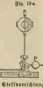
Stellvorrichtung.
