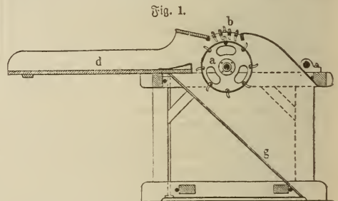
Stiftdreßmaschine.
