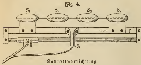
Kontaktvorrichtung.
