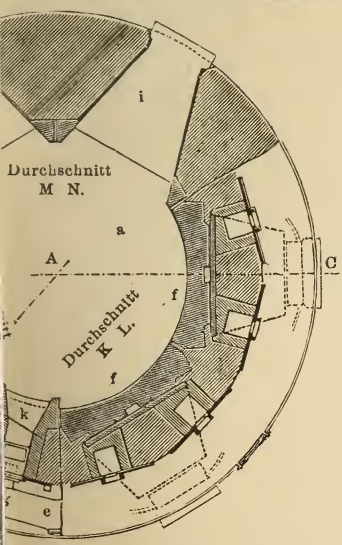
Westmans Gasrösten.
