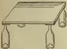
Isolierschemel.
