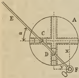
Ellipsenzirkel.
