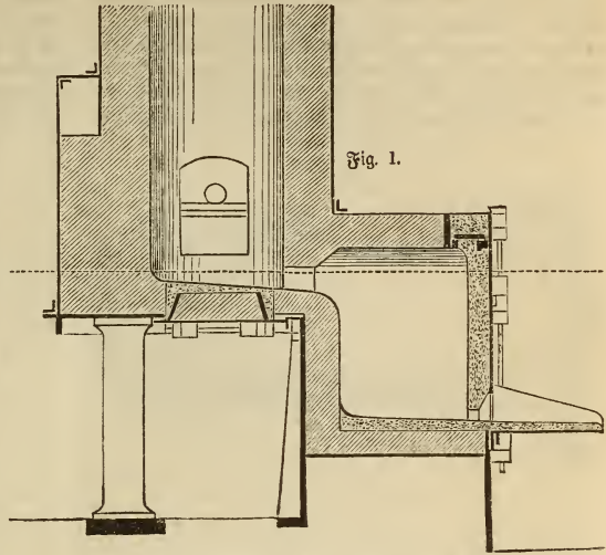
Rigar's Kupolofen. Längendurchschnitt.
