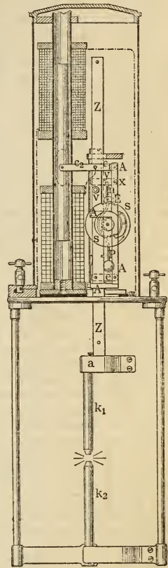
Differentiallampe von Hefner-Alteneck. Durchchnitt.
