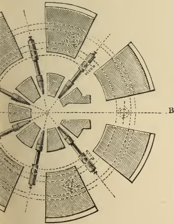
5. Büttgenbachs Hochofen.
