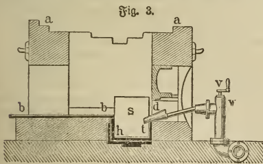
Früschfeuer.
