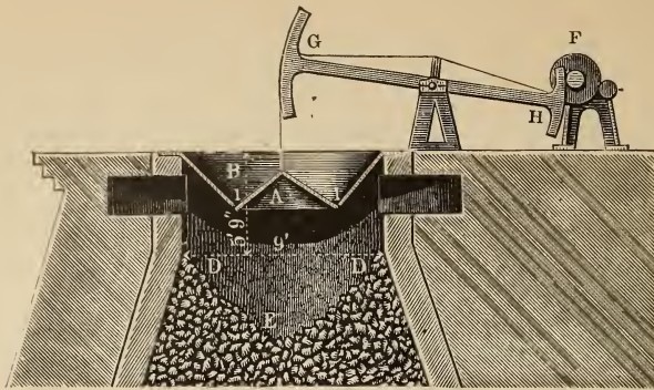
Fig. 8. Parry'scher Trichter.
