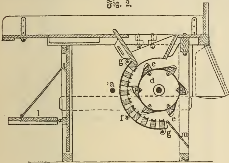
Schlagleistendreschmaschine.
