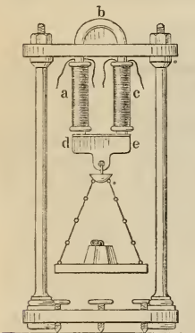
Hufeisenförmiger Elektromagnet.
