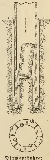
Diamantbohrer
