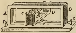
Elektrodynamischer Rotationsapparat.
