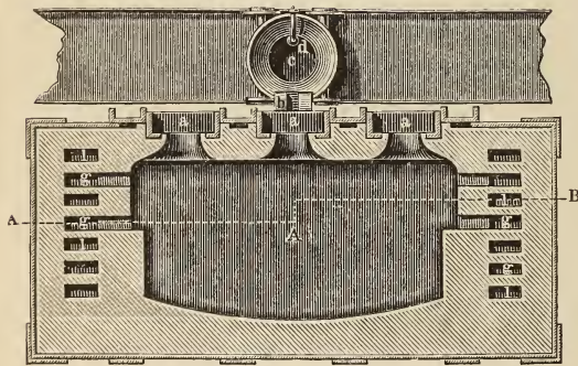
Fig. 27. Siemens-Martin-Ofen.
