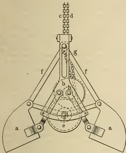
Erzfavator von Voth.
