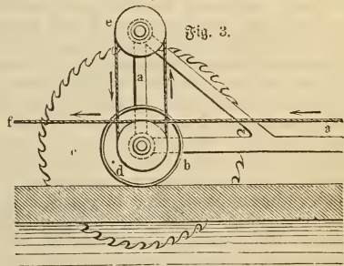
Vorderansicht. Fig. 2 und 3. Dampfispflug.
