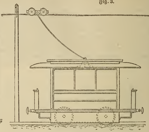
Fig. 2 u. 3. Wagen der elektrischen Eisenbahn bei Charlottenburg.
