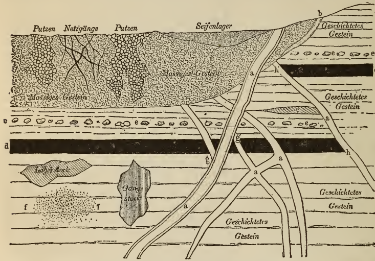
Schematische Darstellung von Erzlagerstätten.
