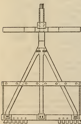
Schachtbohrer.
