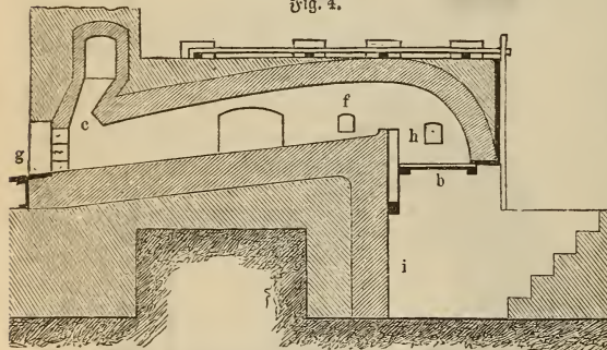
Flammofen. Längendurchschnitt.
