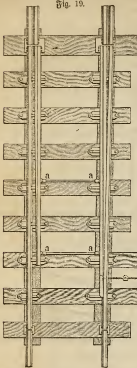
Gleichzeitige Zungenbewegung durch Schubstangen.
