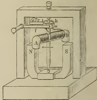
Elektromagnetisches Maschinen von Ritchie.
