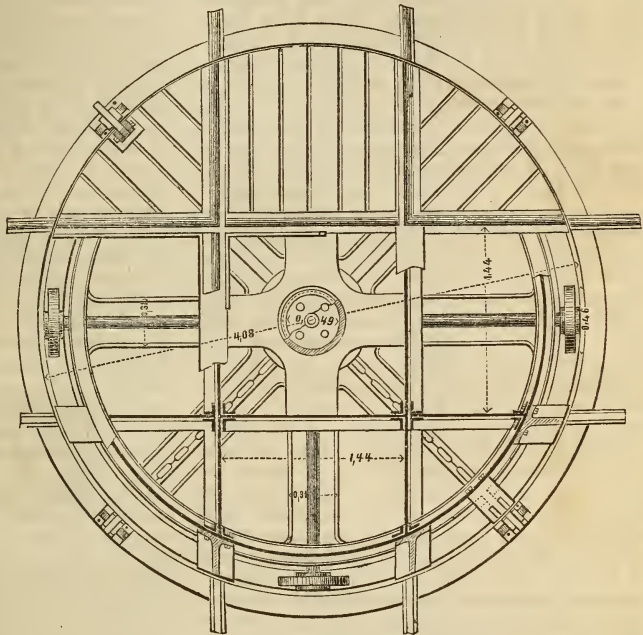
Drehscheibe der Österreichischen Südbahn.
