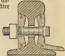
Fig. 6 starke, Fig. 7 schwache Laschen.
