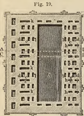
Fig. 18-20. Gaszementstahlöfen.
