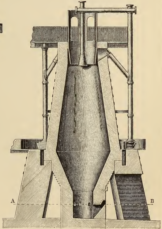
Fig. 4. Büttgenbachs Hochofen.
