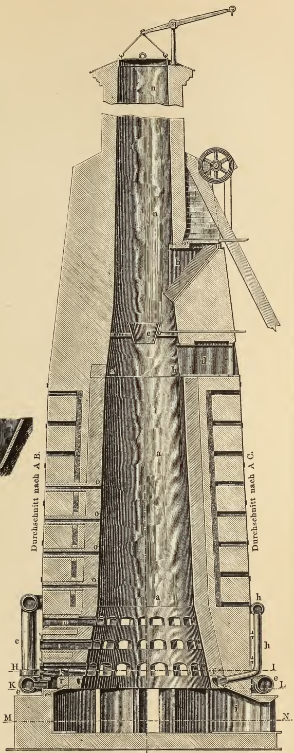
Fig. 1. Westmans Gasrösten.
