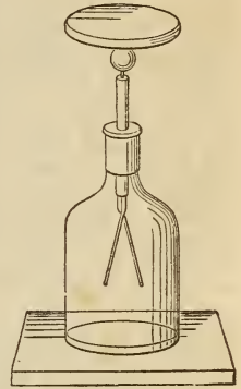
Goldblattelektroskop.
