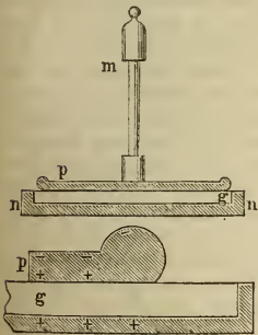
Elektrophor.
