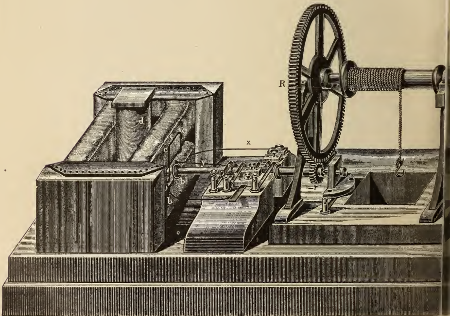
Fig. 2. Störers' elektromagnetische Maschine.
