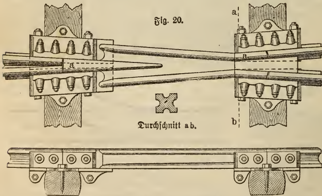
Herzstücke aus Gußstahl zu Weichen.
