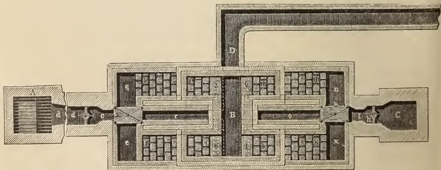
Fig. 23. Siemens' Gußstahlöfen mit Regeneratoren.
