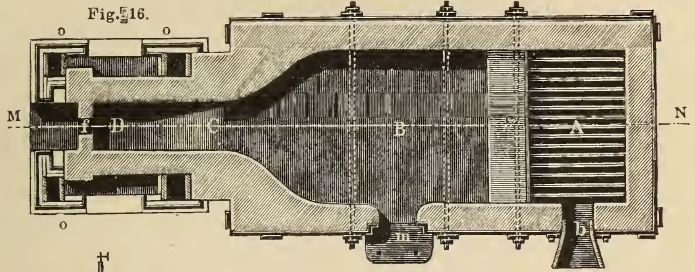
Fig. 15, 16. Schweißofen.
