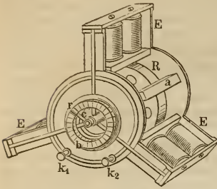
Elektromagnetischer Radmotor von Ruhlo.
