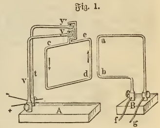
Ampèresches Gestell.
