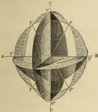
Modell der Wellenfläche der zweiachsigen Kristalle.
