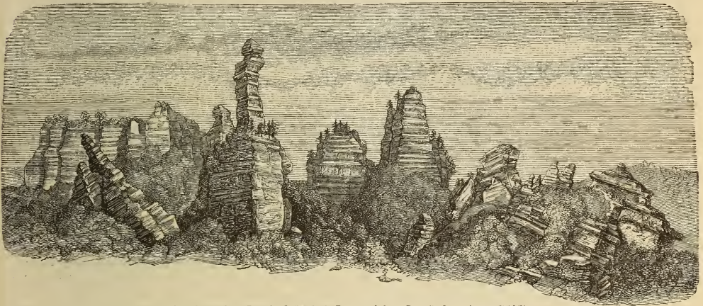
Erosion im Kreidefeld bei Saermi im Kaukasus (nach Abich).
