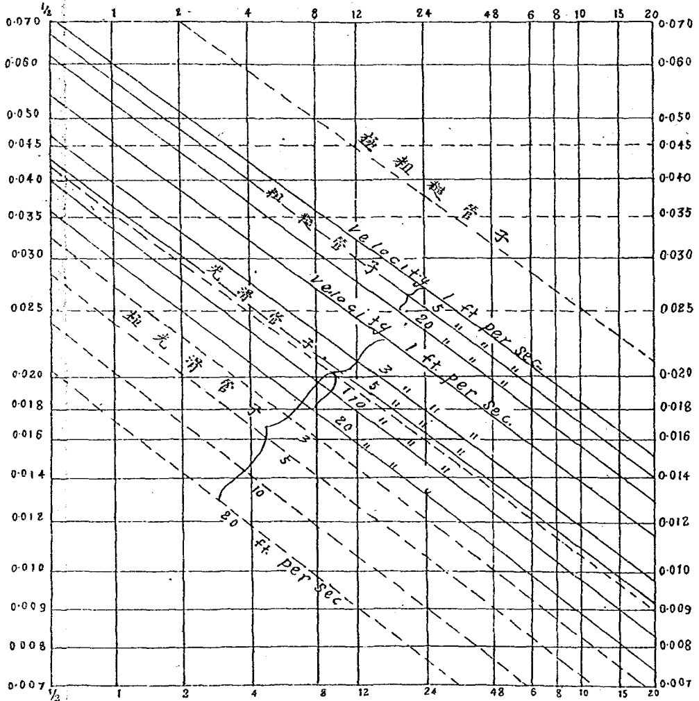
第八圖 圓管阻力係數之數值
