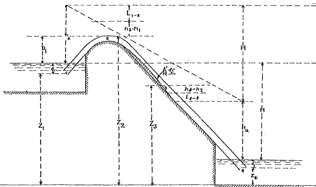
第二圖 强大絕對水頭而管峰不被下游水柱淹沒者
