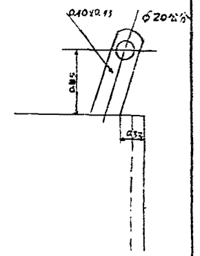
閘耳詳圖 1/50
