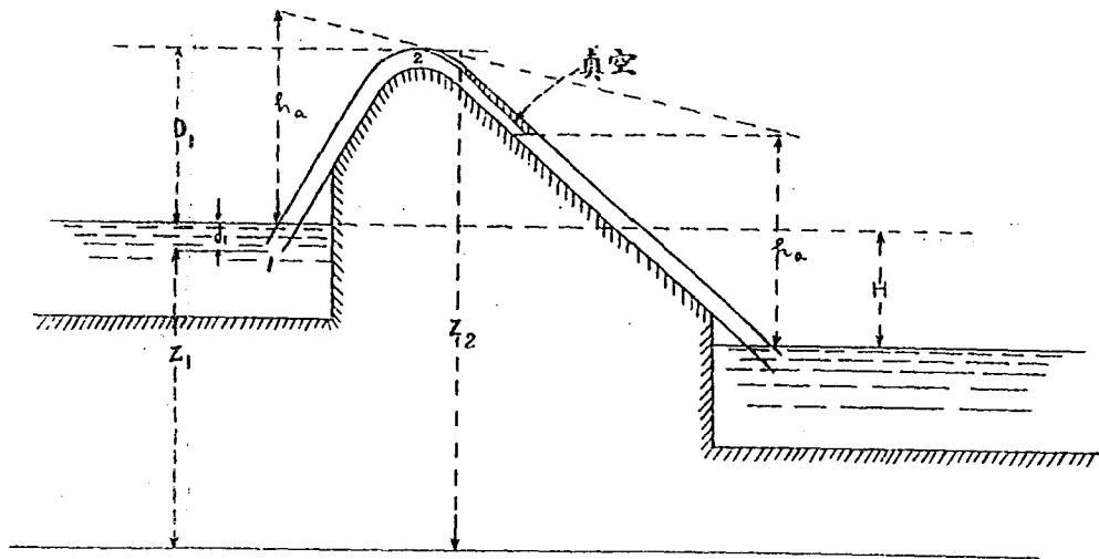
第一圖 微小絕對水頭而管峯不被下游水柱淹沒者
