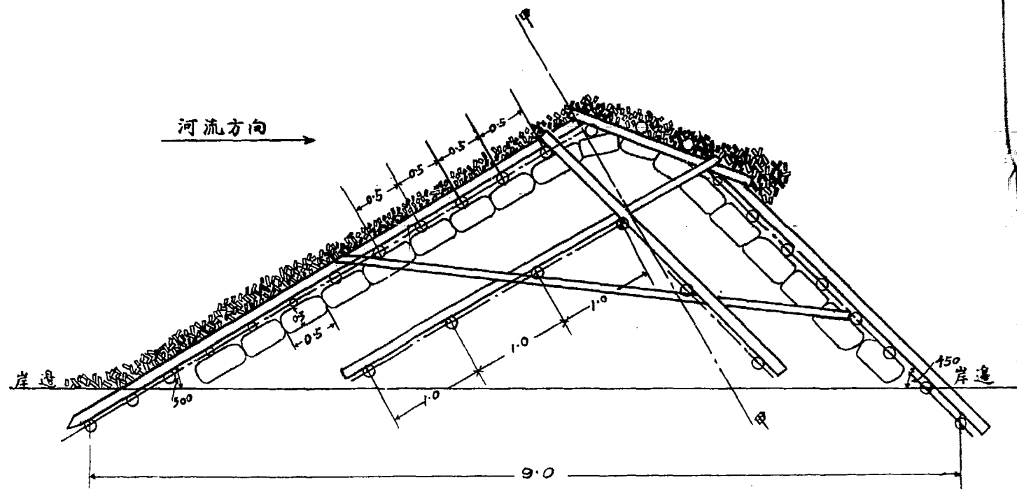
衛河險工碎磚挑水堤標準圖
