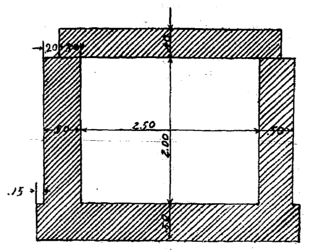
斷面 CD
