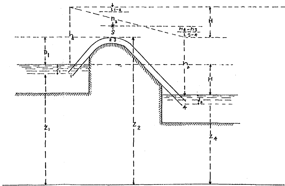
第四圖 强大絕對水頭而管峯被下游水柱淹沒者
