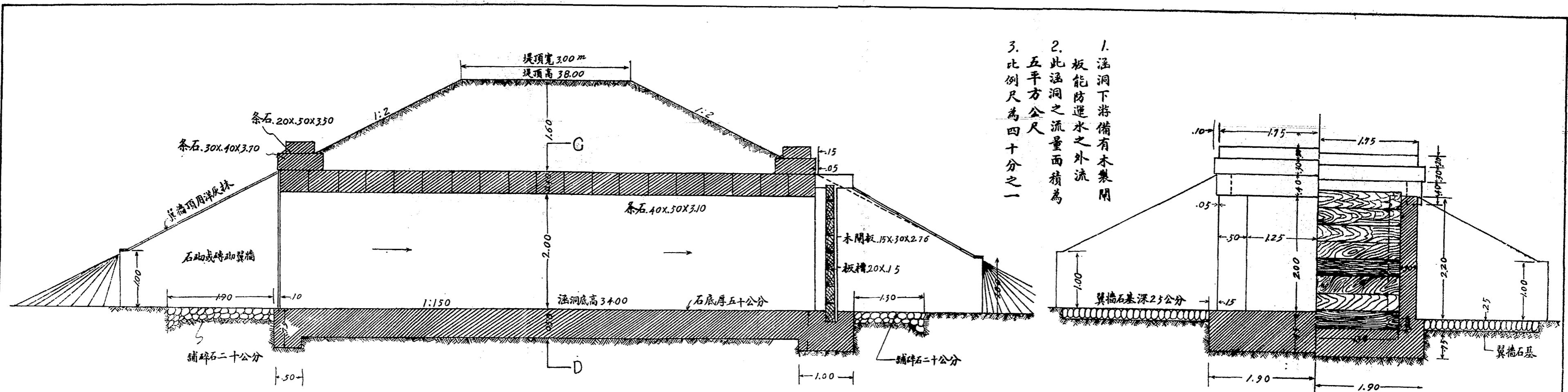
縱斷面 AB
