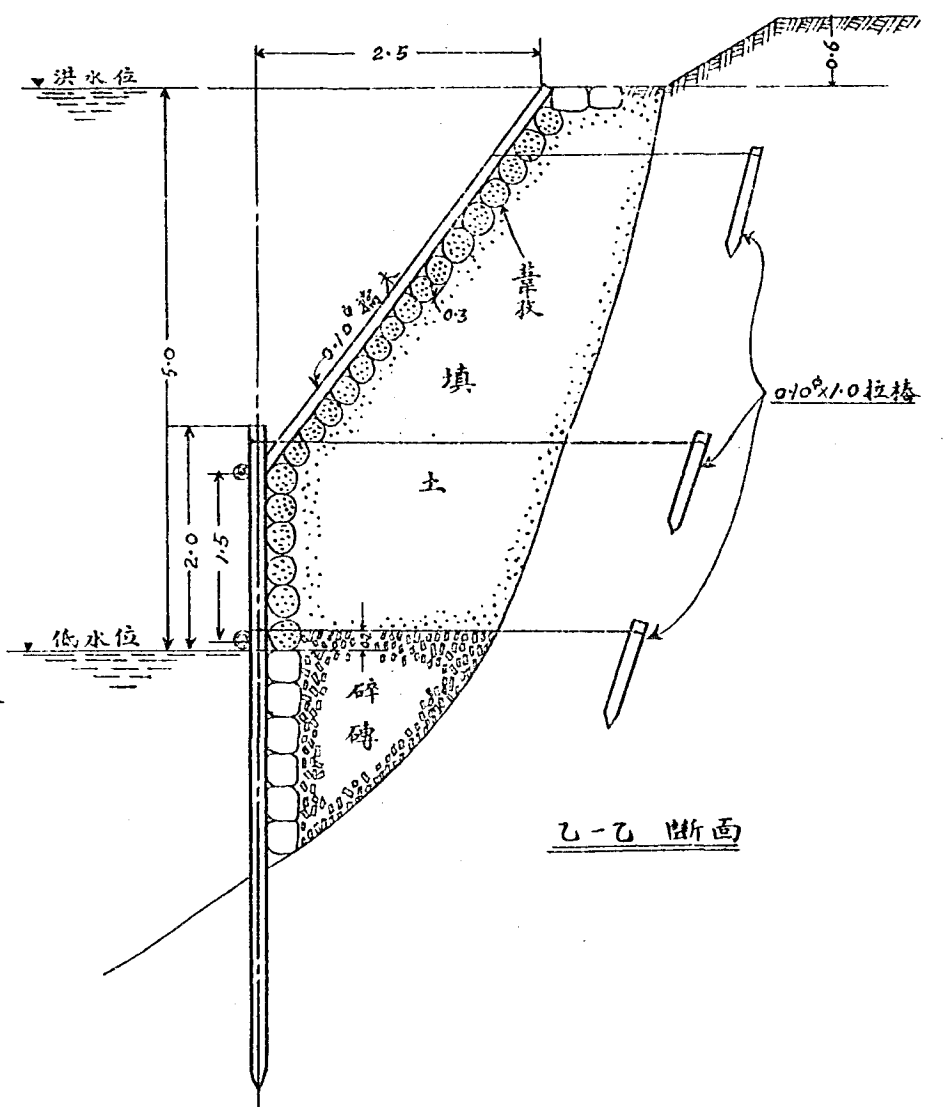
衛河險工碎磚加料挑水堤標準圖 比例尺: 1:50
