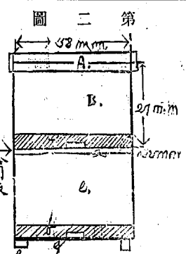
圖二第 A、示上箱箱蓋 B、示上箱箱身 C、示門木 D、示合同板之位置 E、下箱箱身 F、示門木 G、示下箱箱底 H、示墊箱木石
