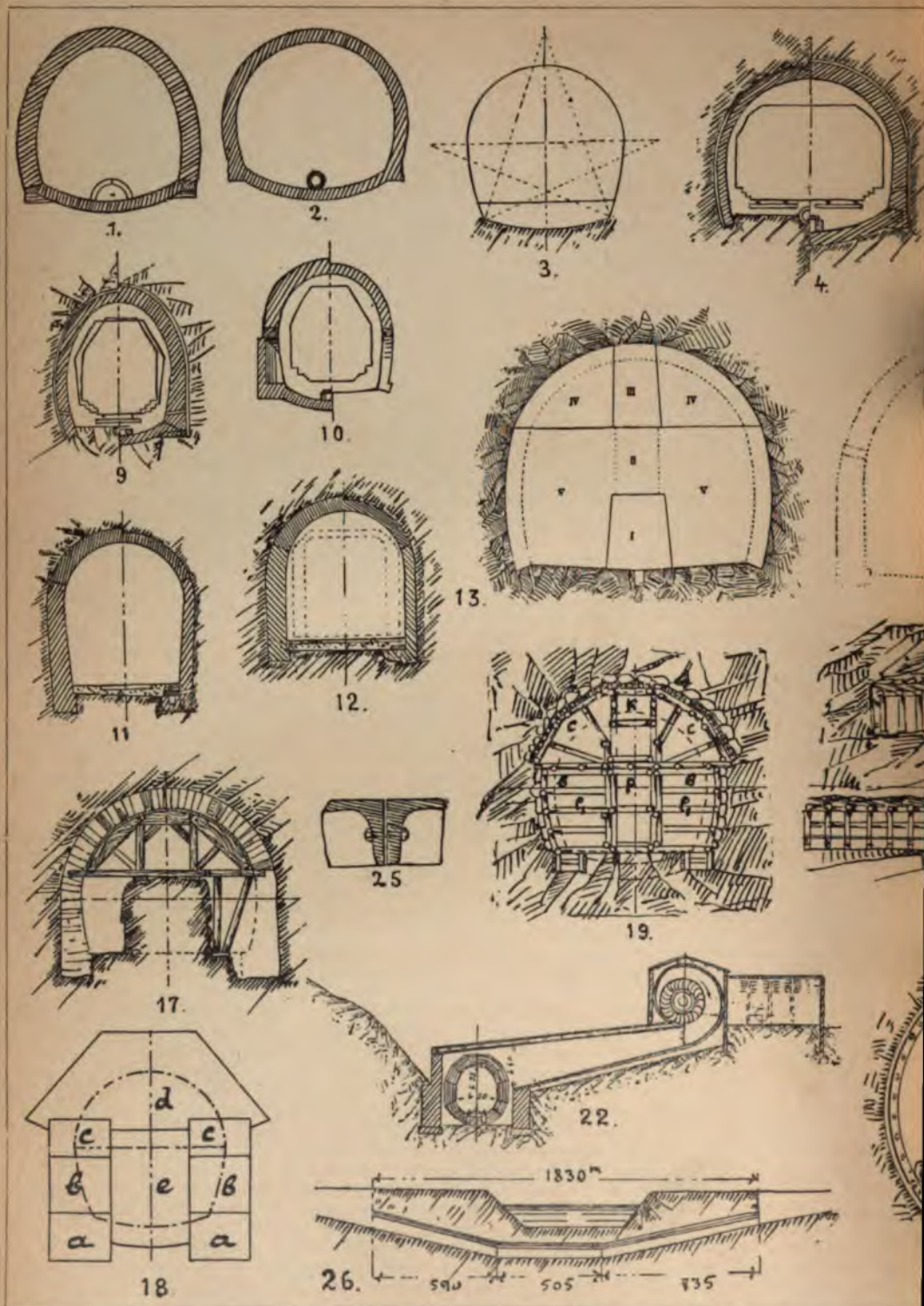
1. Блечинглейскій Т. 2. Северскій Т. 3. Профиль Т. жел. дор. Земмерингъ. 4. Нормальный профиль, принятый въ Германіи. 5. Профиль для Т. въ одинъ путь. 10. Однопутный Т. Львовскійхъ жел. дор. въ Русси. 11. Профиль Т. вая половина—обдѣлана въ скалистой породѣ, дѣвая въ мерели и обломочной породѣ. 13. Раздѣленіе профилей Т. 14. Ігійскимъ способомъ. 18. Схема послѣдовательнаго хода работъ по вѣнскому способу. 19 и 20. Австрійскій способъ. 21. Поперечное сѣченіе чугуина Ватерло-Сити (7 сегментовъ), IV. Т. коллектора въ Клинки (5 сегментовъ) 25. Способъ скрѣпленія сегментовъ. 26. Продольное сѣченіе (для про...
