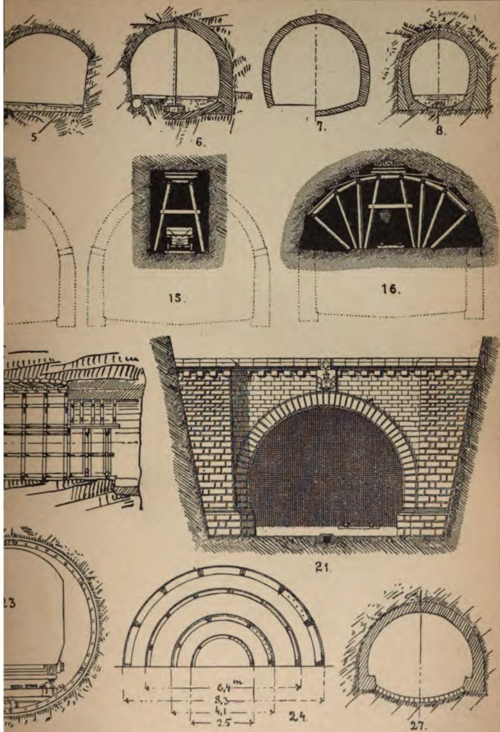
5 и 6. Профили С.-Готтардского Т. 7. Профиль прусского Т. 8. Т. жел. дороги Озарина-Штейердорф. ж. дор. Сквалга, в морей и обломочной породе. 12. Профиль Т. зубчатой жел. дор. на гору Горнерграт. Пра- вья. 15. Разработка ключевой штольни. 16. Дальнейшая разработка бельгийским способом. 17. Обделка бель- гий из Т. Владикавказской жел. дор. 22. Вентиляция по системѣ Саккардо. 23. Поперечное сѣчение Т. съ чугун- ными ильготорыжъ Г.—I Влекувельскій Т (14 сегментовъ). II. Сенъ-Клерскій Т (13 сегментовъ). III. Т. жел. дор. въ Т. подъ р. Сенъ-Клеръ, форть Гуронъ въ Соедин. Штатахъ Сѣв. Америки. 27. Т. подъ железнодорожною
