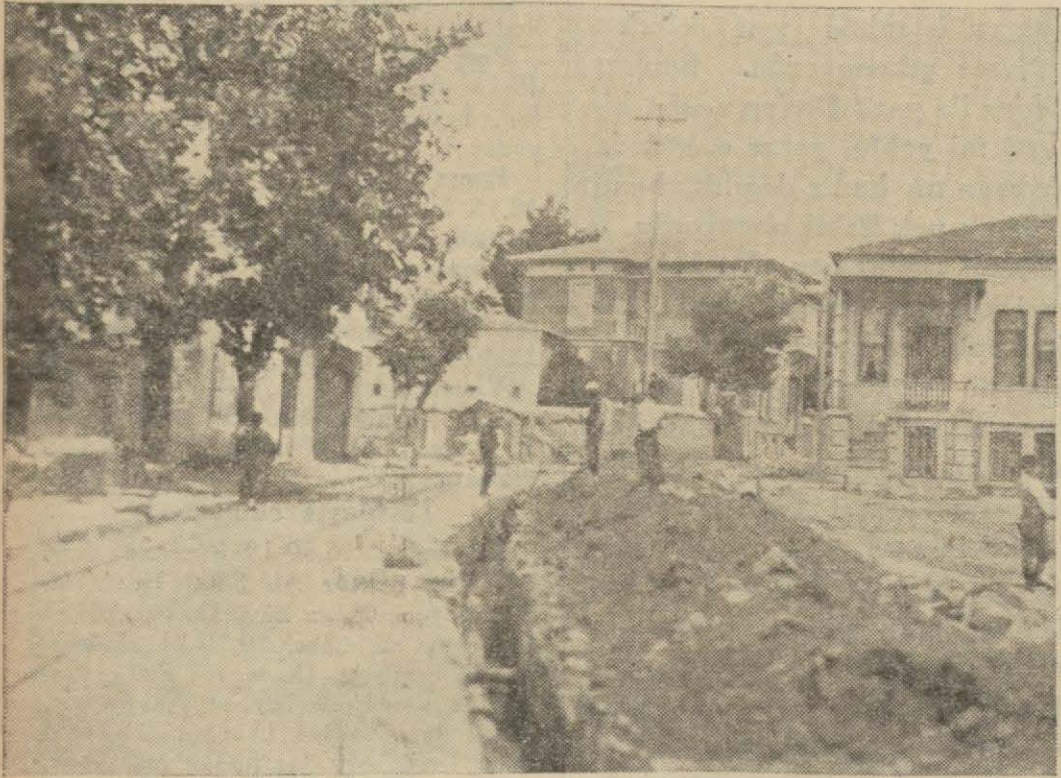
Boru ferşi ameliyatı
