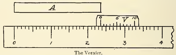
The Vernier.
