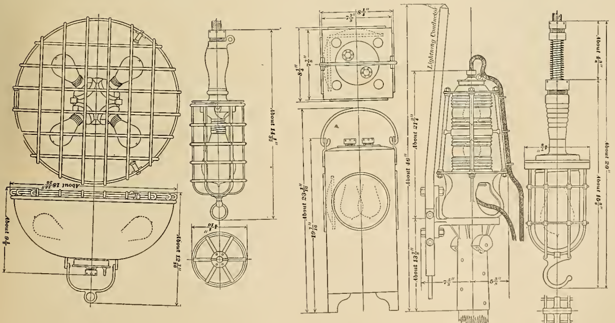
Cargo Reflector.
