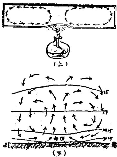
第一四圖 上圖表明水燒熱之後，在鍋裏流動的情形；下圖表明地球上的熱空氣，從赤道上升，分向南北兩極流去的情形。
