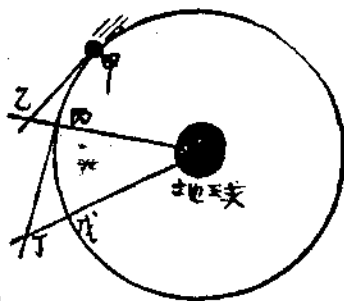
第十三圖 看了這圖，就知道，月亮實在是時時刻刻向地球落下來。
