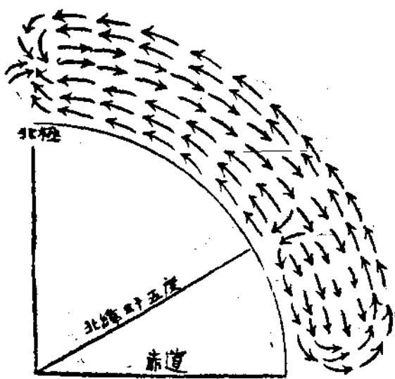
第一三圖 從赤道上升的空氣，向北極流去的情形。
