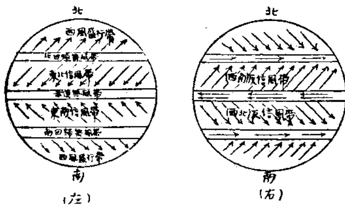
第一二圖 左圖表明靠近地面的大氣流動的方向；右圖表明天空大氣流動的方向。
