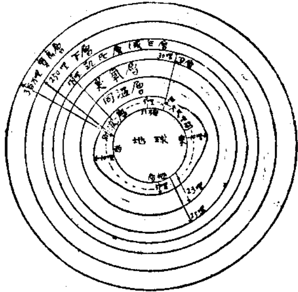
第一圖 地球的各層
