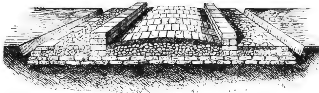
Фиг. 4. Разрѣзъ уличной мостовой у древнихъ римлянъ.
