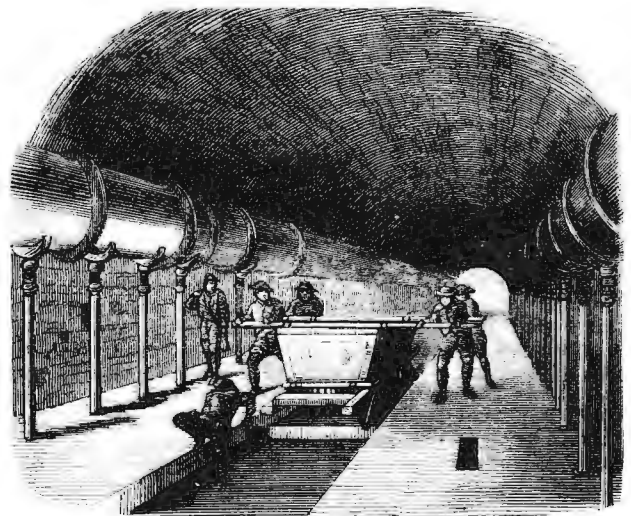
Фиг. 6. Большая подземная очистительная машина.
