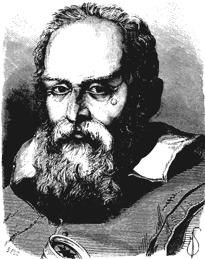
Галилей.
