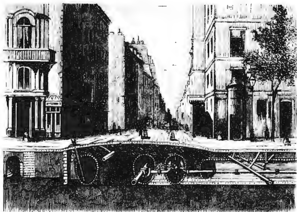
Фиг. 5. Разрѣзъ современной мостовой.
