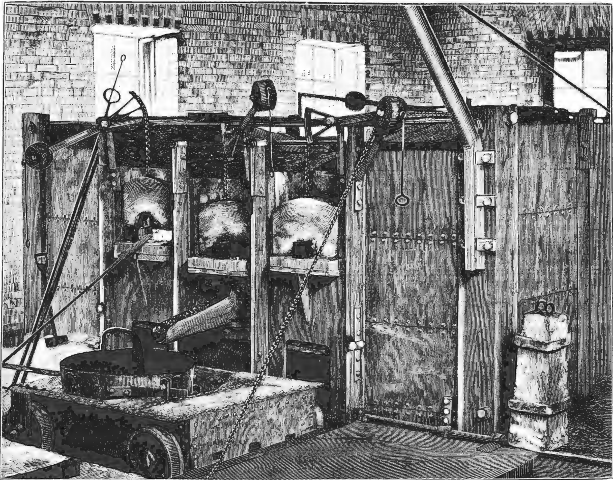
Сормовскій сталелитейный заводъ. Видъ печи для плавки стали по способу Сименсъ-Мартена. Съ фот. Карелина въ Н. Новгородѣ грав. Рашевскій.
