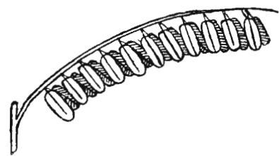
Фиг. 14. Паденн барометра.
