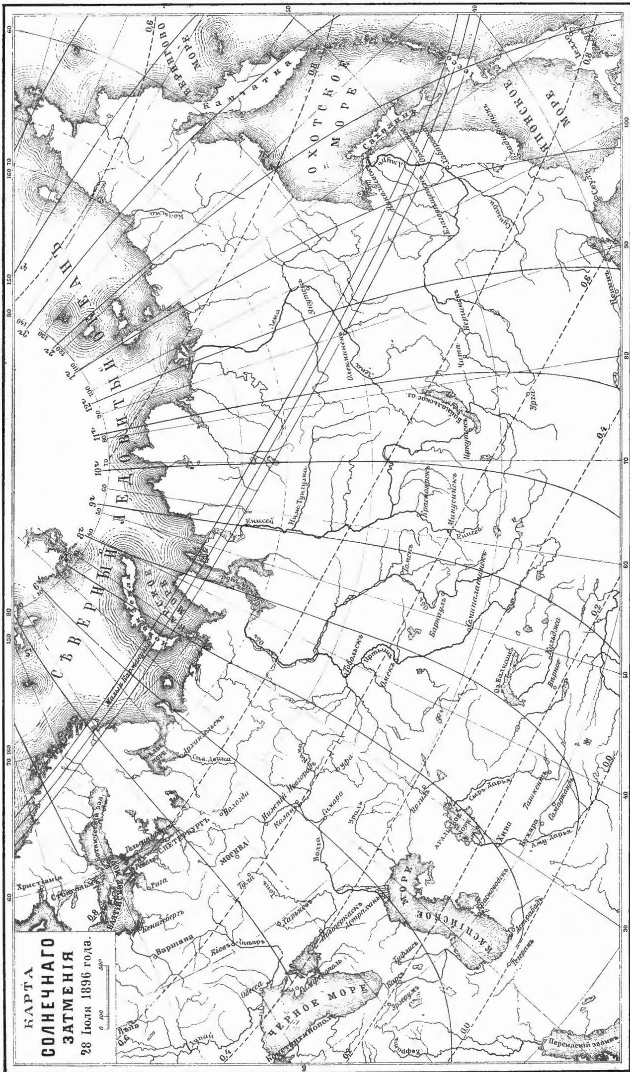
Полное солнечное затмение 28 июля 1896 года.
