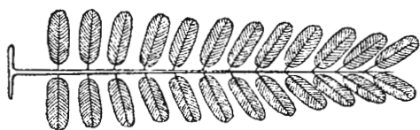
Фиг. 5. Перемѣнно, съ начинающимся вѣтромъ.
