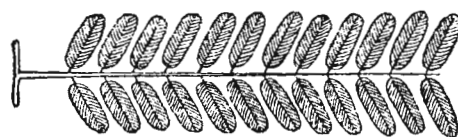
Фиг. 6. Перемѣнно и вѣтеръ.
