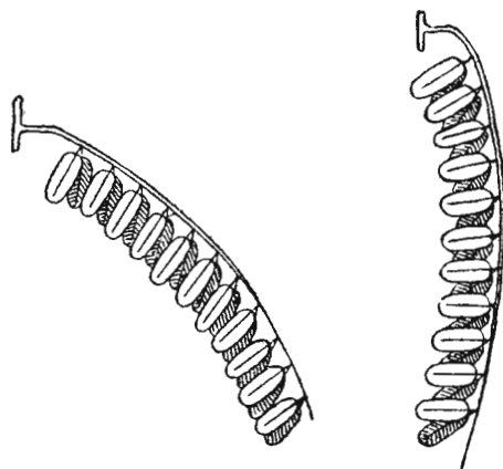
Фиг. 16. Высшее бараметрическое давленн (максимумъ).
