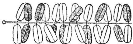
Фиг. 1. Туманъ или тучи.
