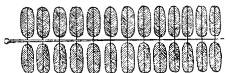
Фиг. 4. Перемѣнно, тихо.
