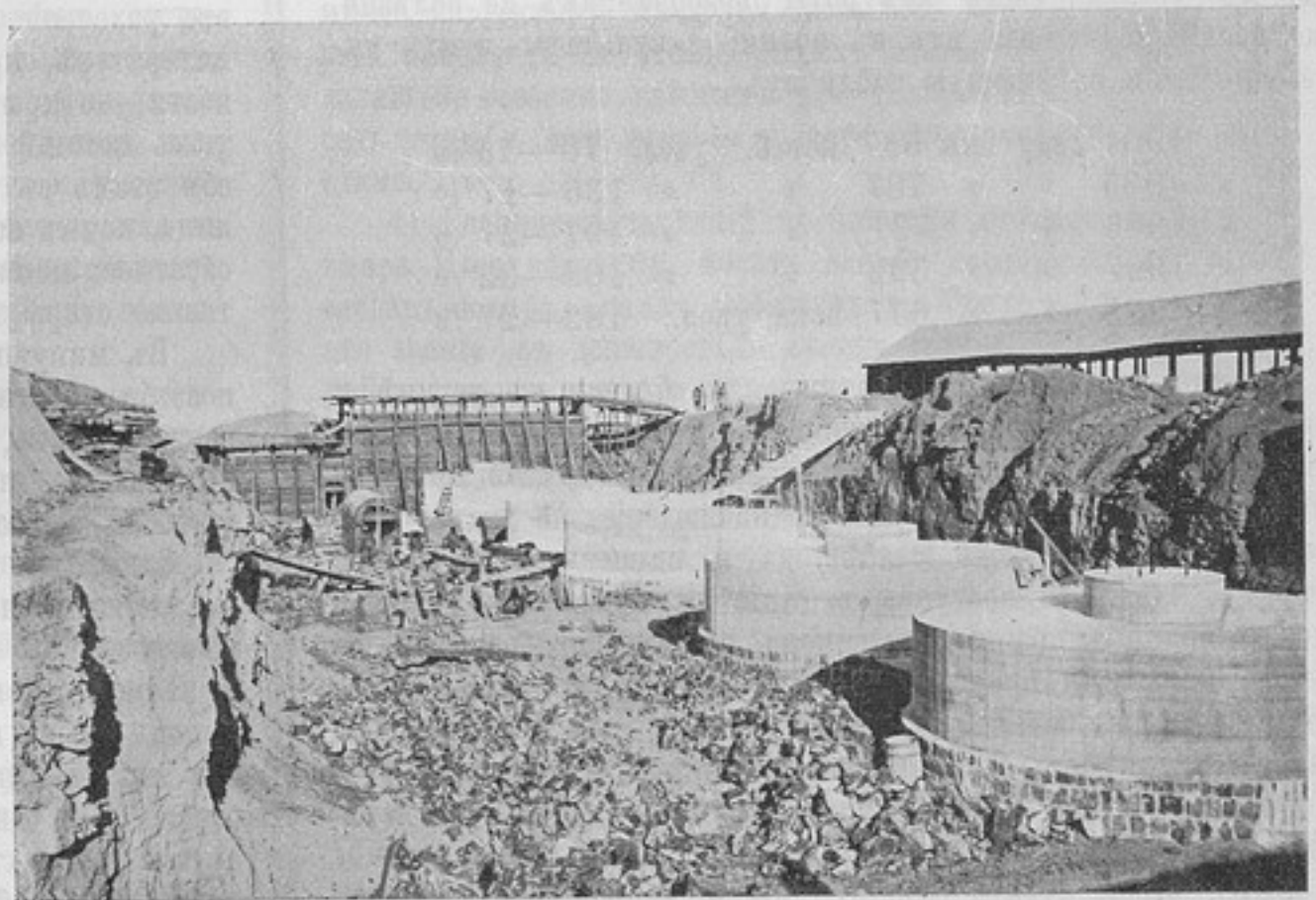
Устройство основаній для установки орудій на береговой батарее. (Изъ книги «Оборона Портъ-Артура»).
