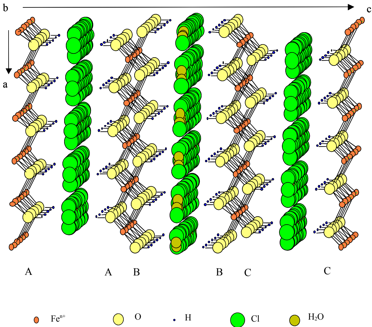
Figure 4 : Structure de la rouille verte GR(Cl)
