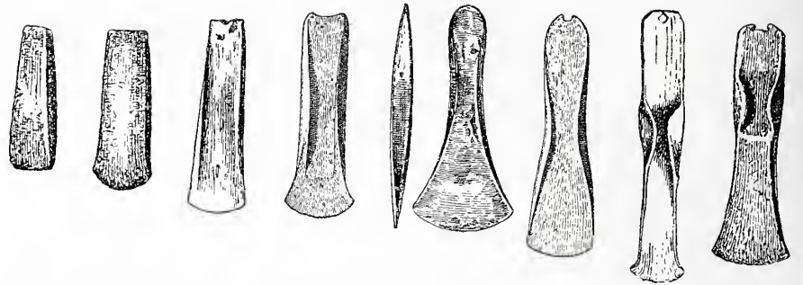
Fig. 8. Die Entwicklung vom Kupferbeil in Steinbeilform bis zur Lappenaxt der späteren Bronzezeit (nach Forrer)
