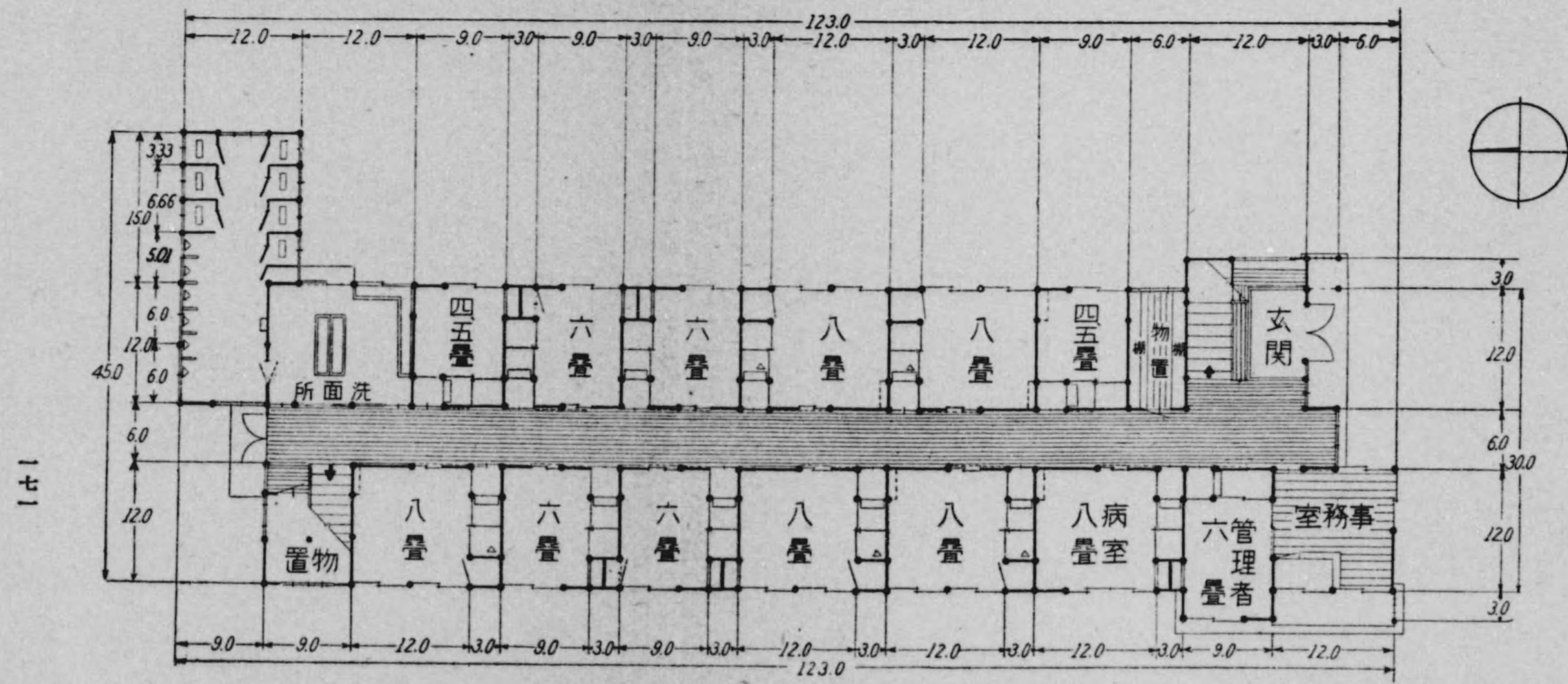
圖面平階一
