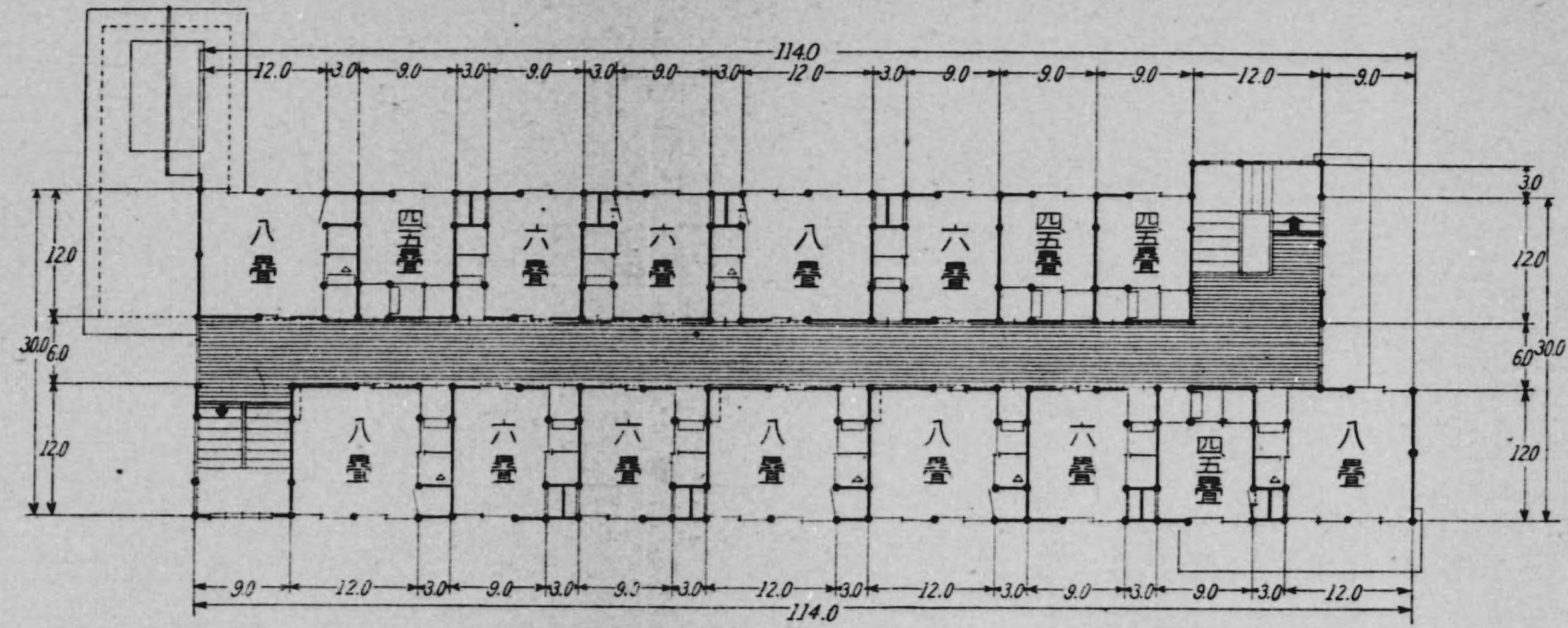
圖面平階二
