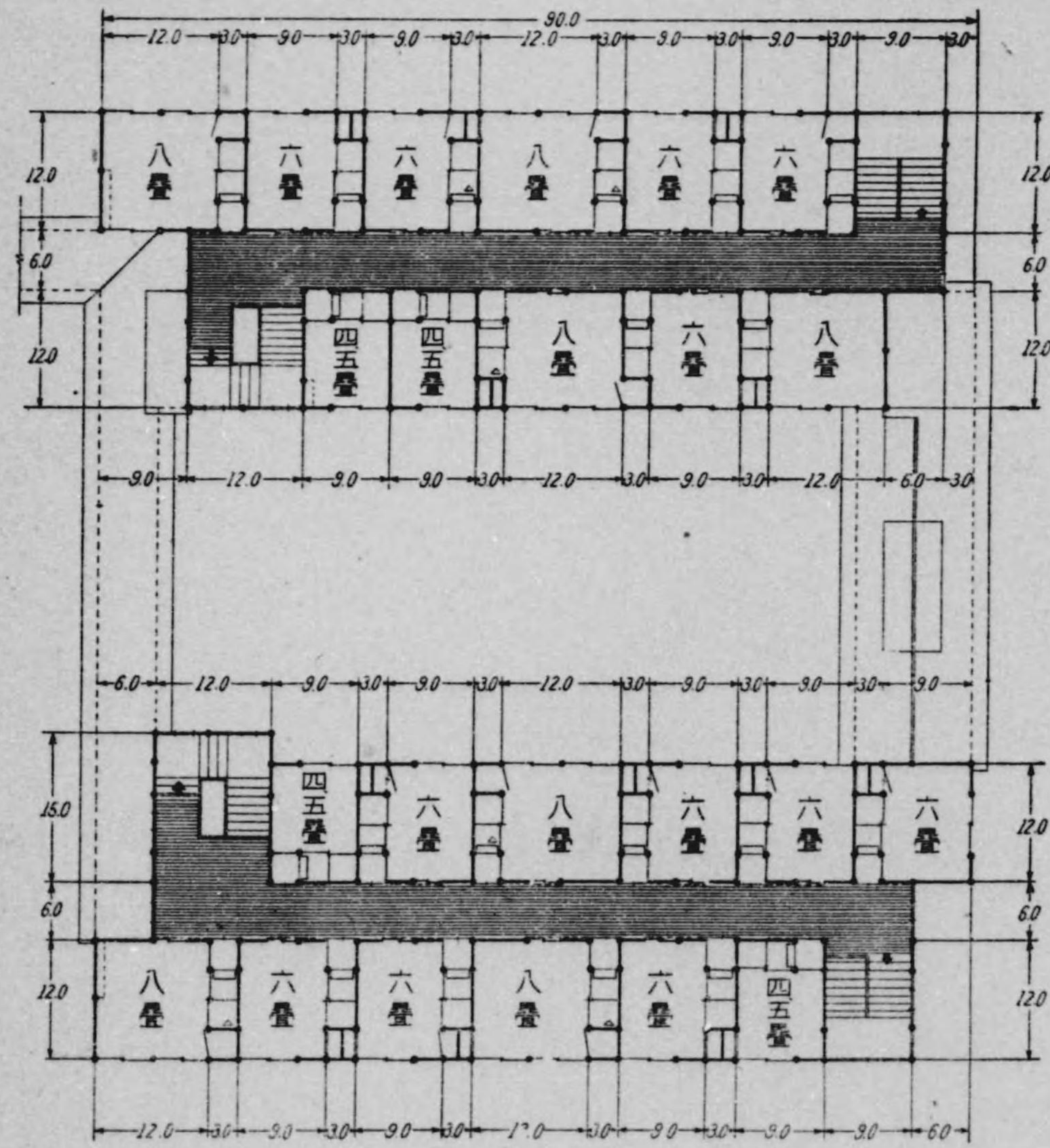
圖面平階二
