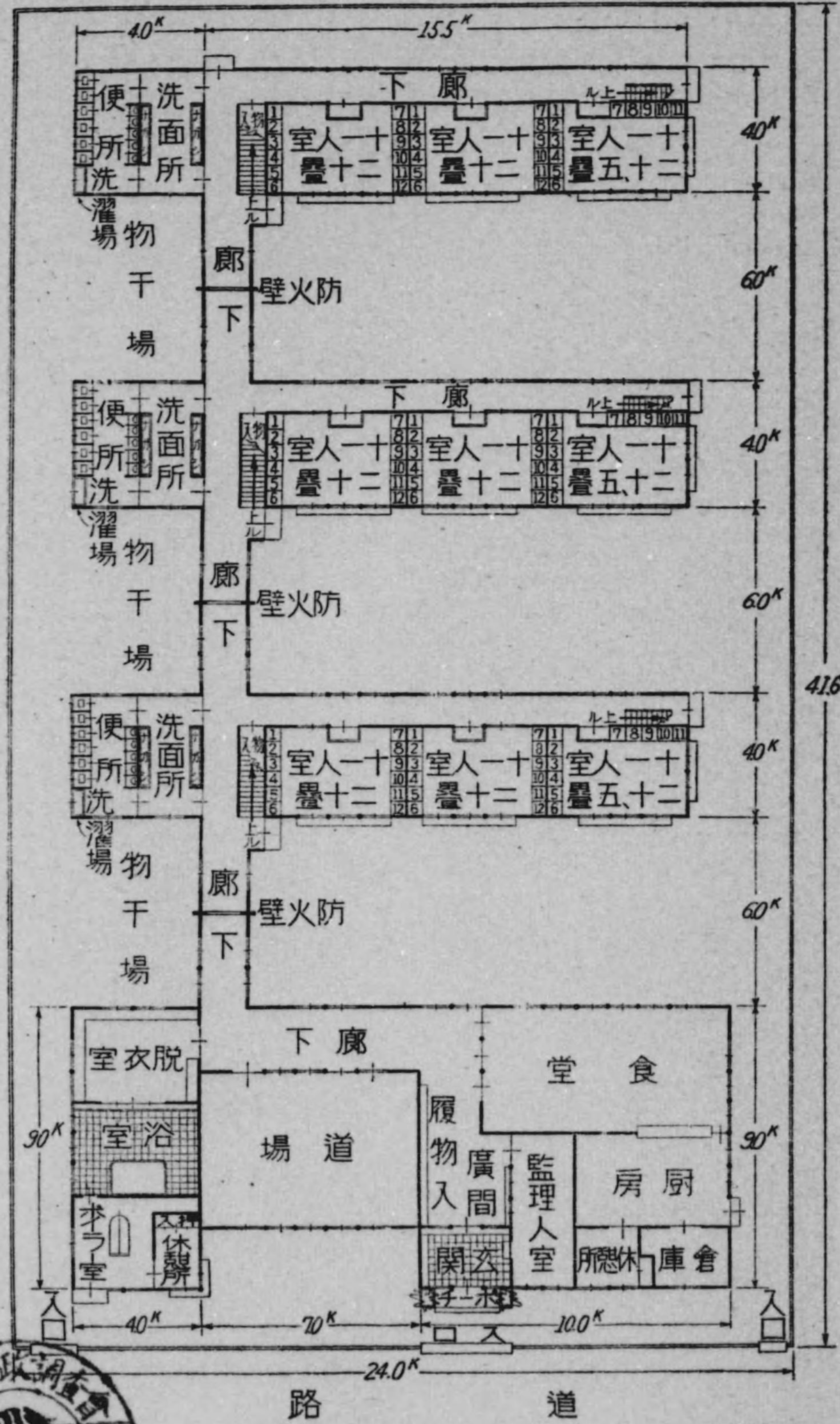
圖 面 平 階 一
