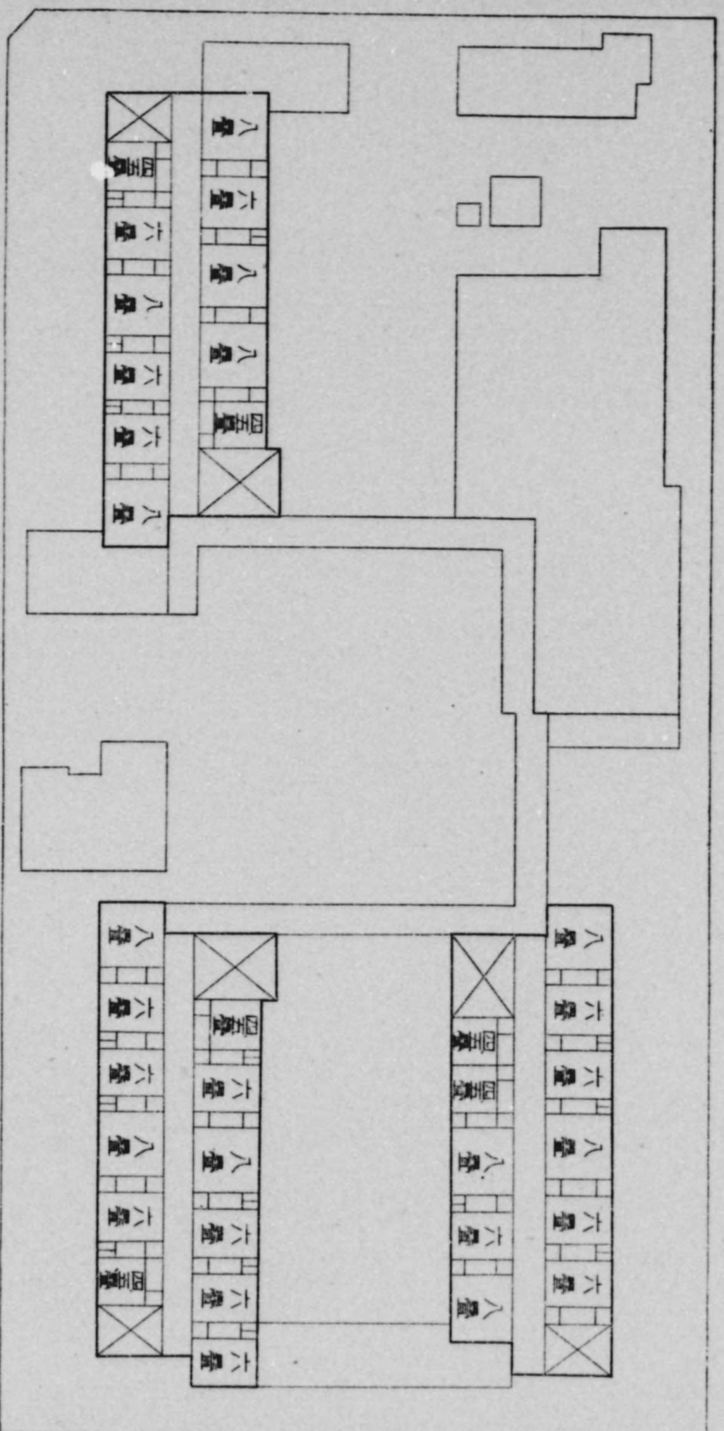
圖面平階二
