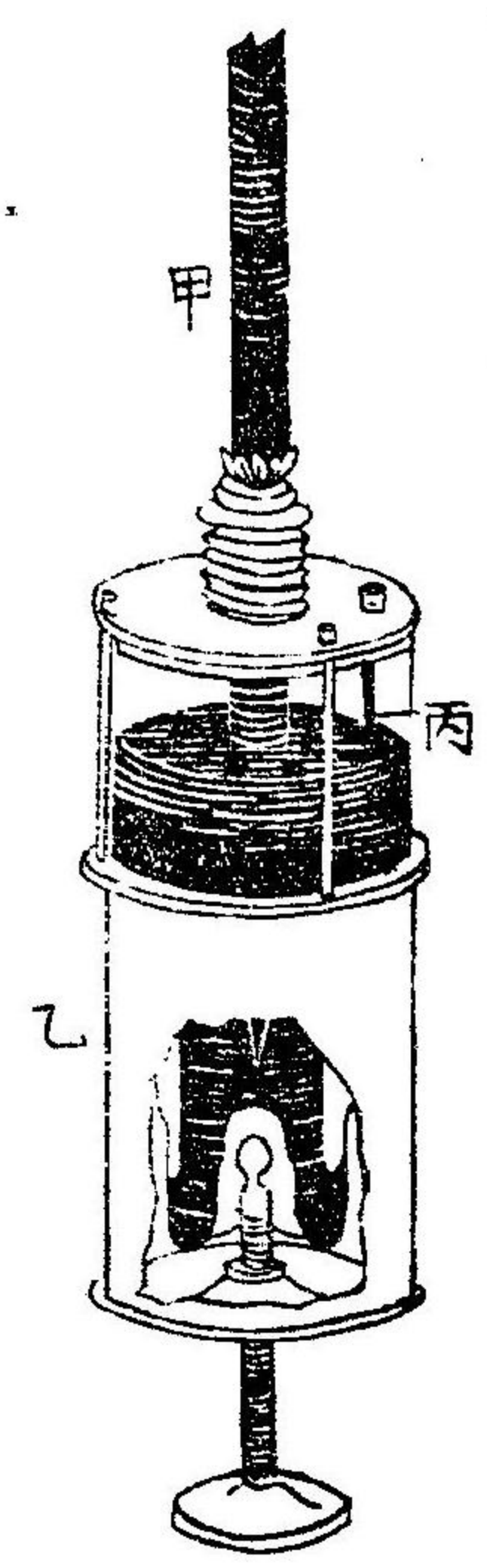
第九十六圖ノ如 シ乃チ「甲」ヲ氣壓表 トシ「乙」ヲ槽トス
