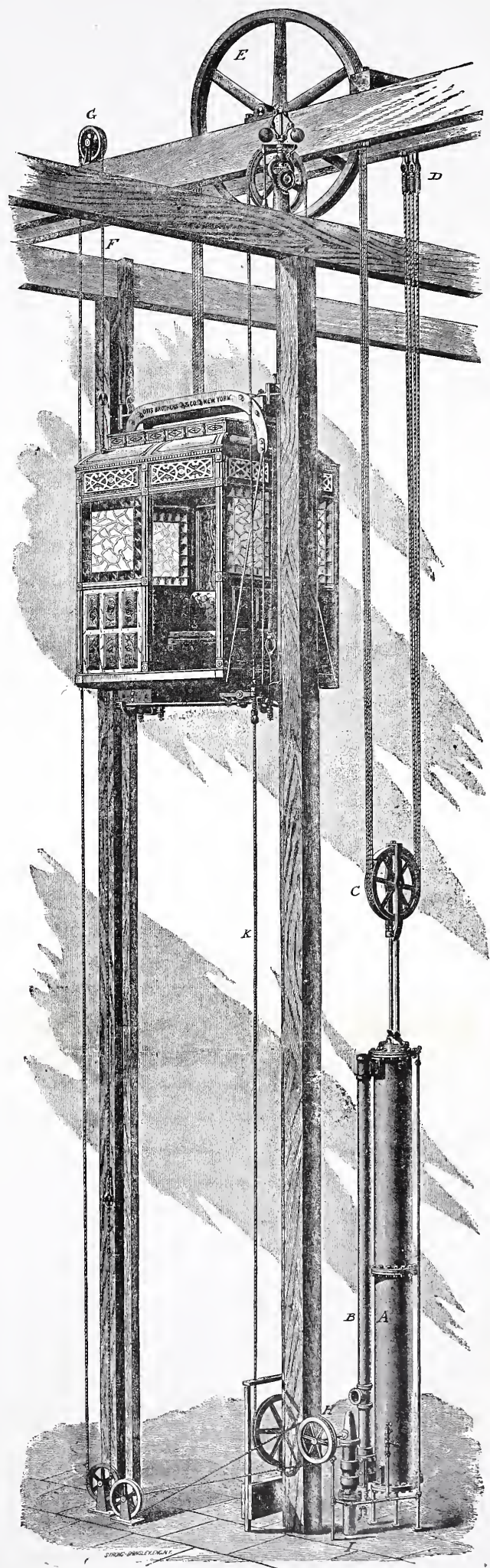
Fig. 1. Algemeene inrichting.
