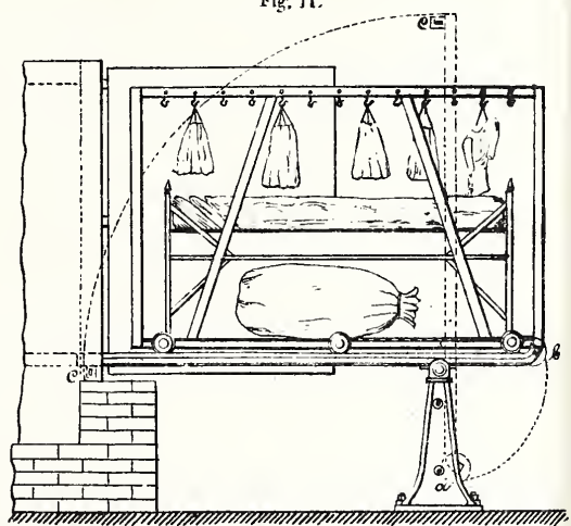
Henneberg's Desinfektor C.
