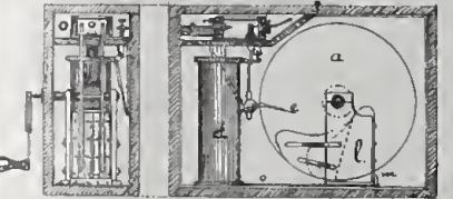
Fig. 14. Platte grond.
