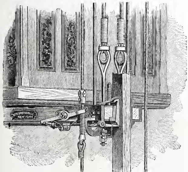
Fig. 5. Veiligheidswig.
