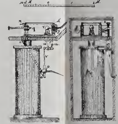
Fig. 16. Condensator met Ontlader.
