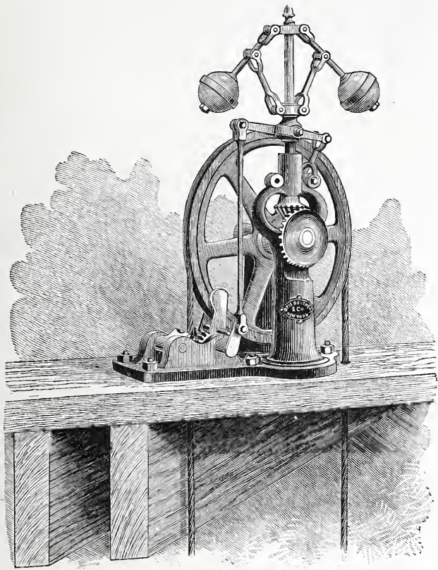
Fig. 4. Snelheids regelaar.
