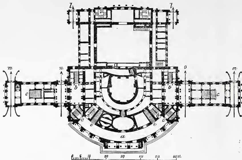
Platten grond van den nieuwen hofschouwburg te Weenen.
