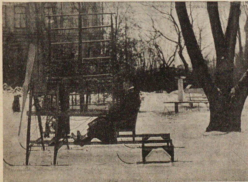
Аэро-сани № 1.
