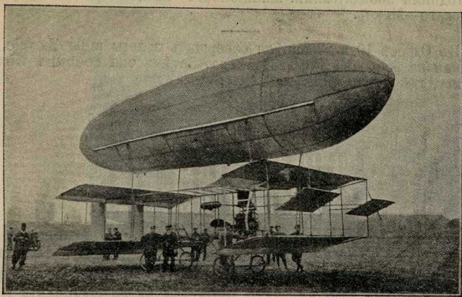
Дирижабль-миксть конструкции Цезаря.
