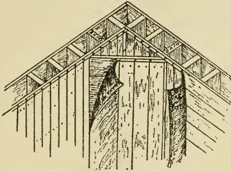
Fig. 23. Corner of rectangular silo. (Whceler.)
