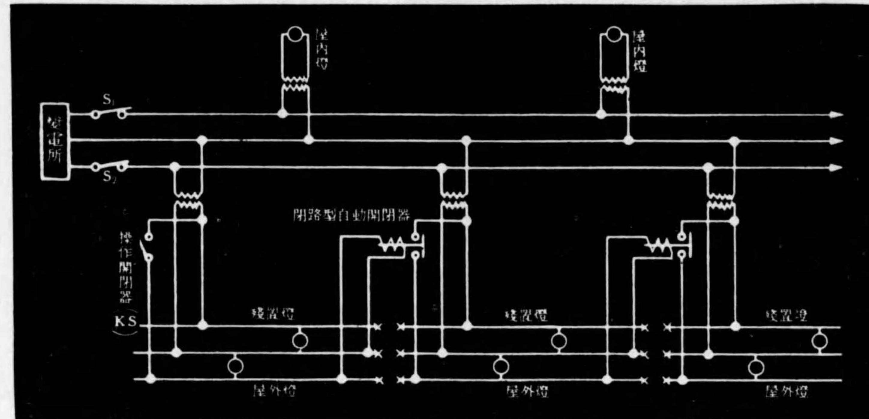
第二圖 三相又ハ單相三線式
