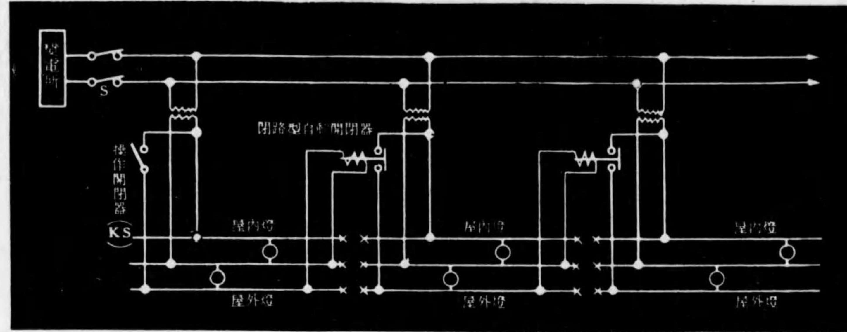
第二圖 三相又ハ單相三線式
