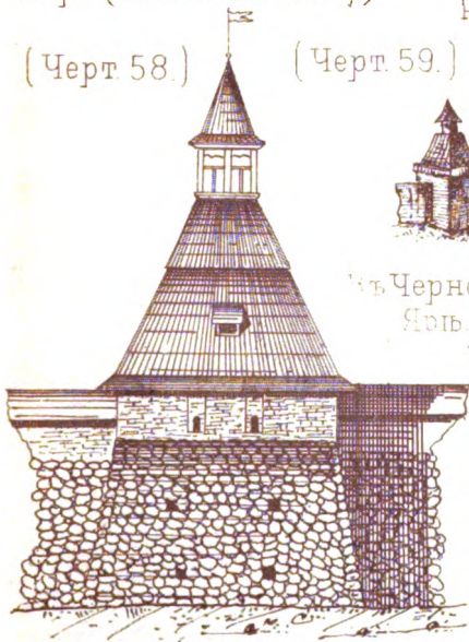
Башня въ Соловецкомъ Монас- тыря (по Ласковскому).
