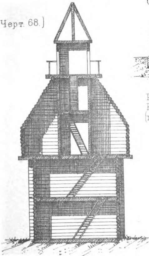
Башня въ г Красноярскъ. (по Ласковскому)
