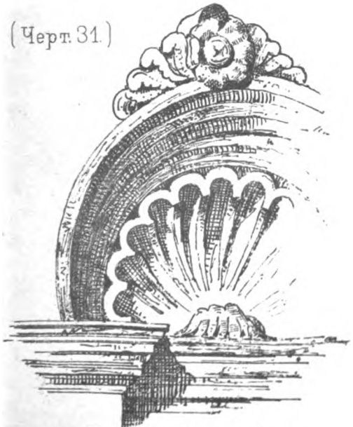
Кокошникъ Архангельскаго собора въ Москвѣ (по Далю)
