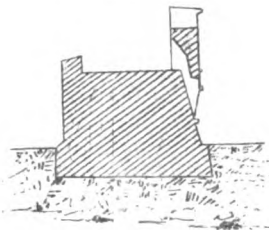
Разрѣзь стѣны Китай-города (по Ласковскому)
