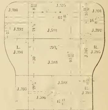
Fig. 14.—Holder Plate.
