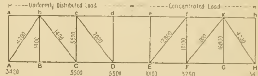
Fig. 2—Stress Diagram.
