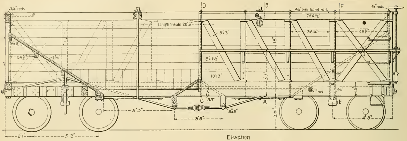
Elevation
