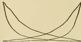
M. E. P., 33.6. M. E. P., 30.3. I. H. P., 196. I. H. P., 184.
