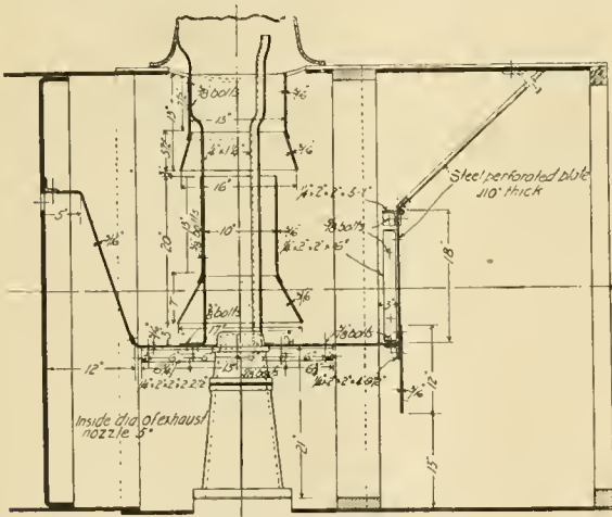
Fig. 1. - Norfolk & Western.
