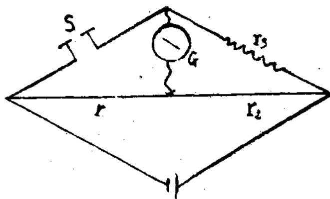
第二圖 尺線電橋
