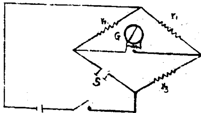
第一圖 惠斯登橋
