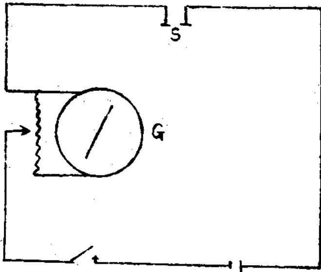
第四圖 簡單電路
