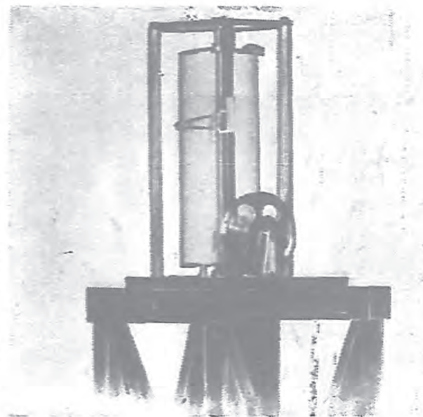
圖示：立式自動手尺，係水利部中央水利 實驗處水工儀器工廠製造，可與瑞士出品 相埒。
