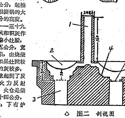
图二 剖视图
