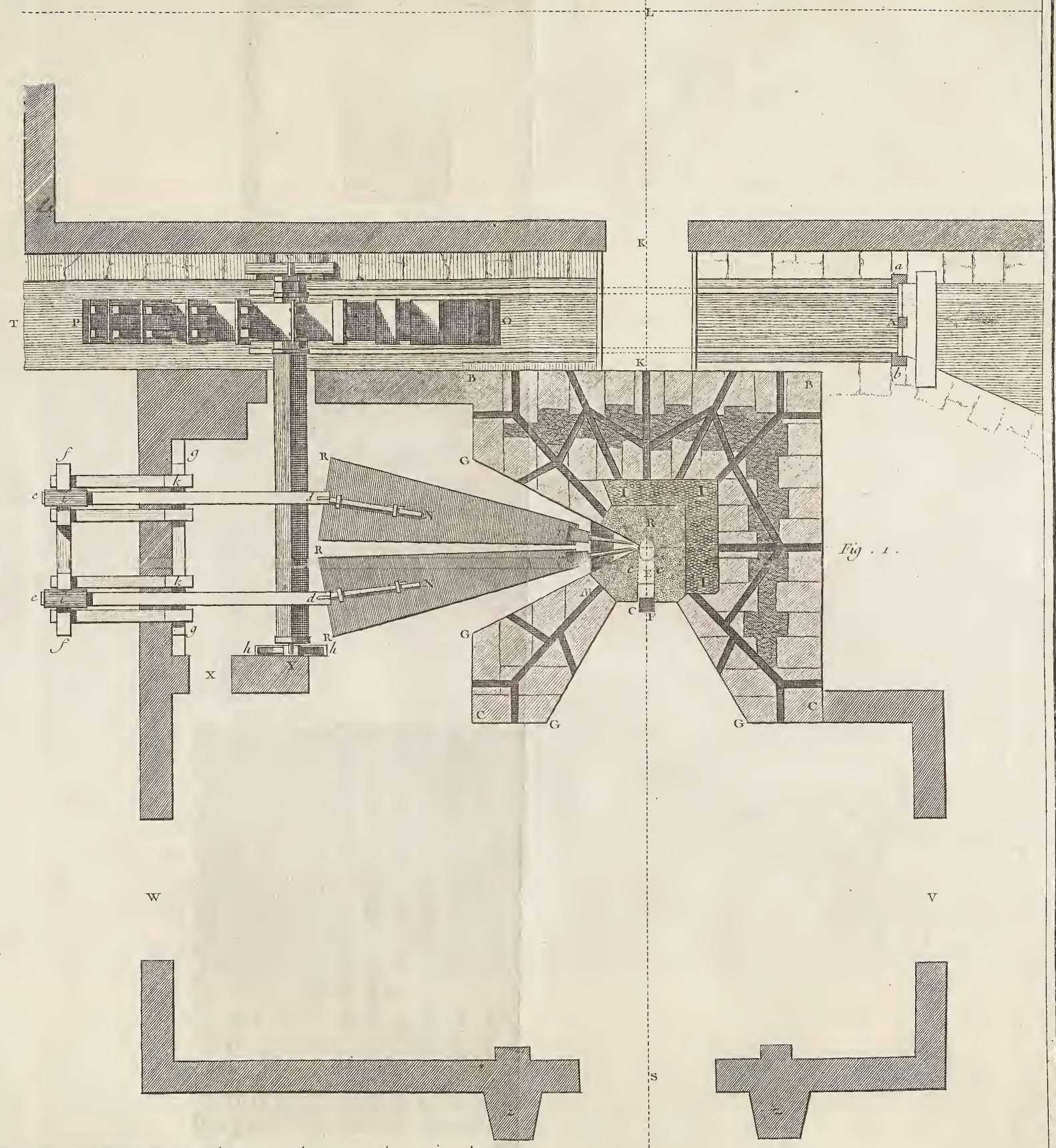
Forges, 2 e Section, Fourneau à Fer, Plan General et Particulier d'un Fourneau.
