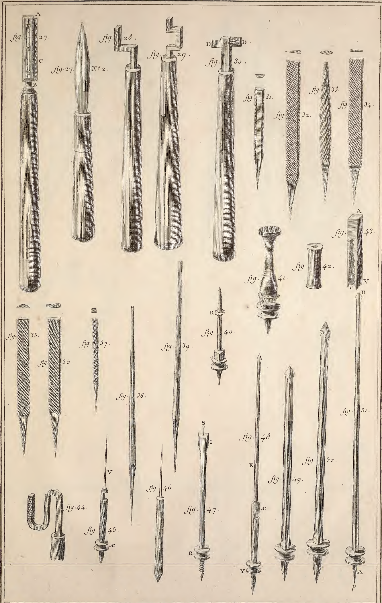
Horlogerie, Différens Outils d'Horlogerie.
