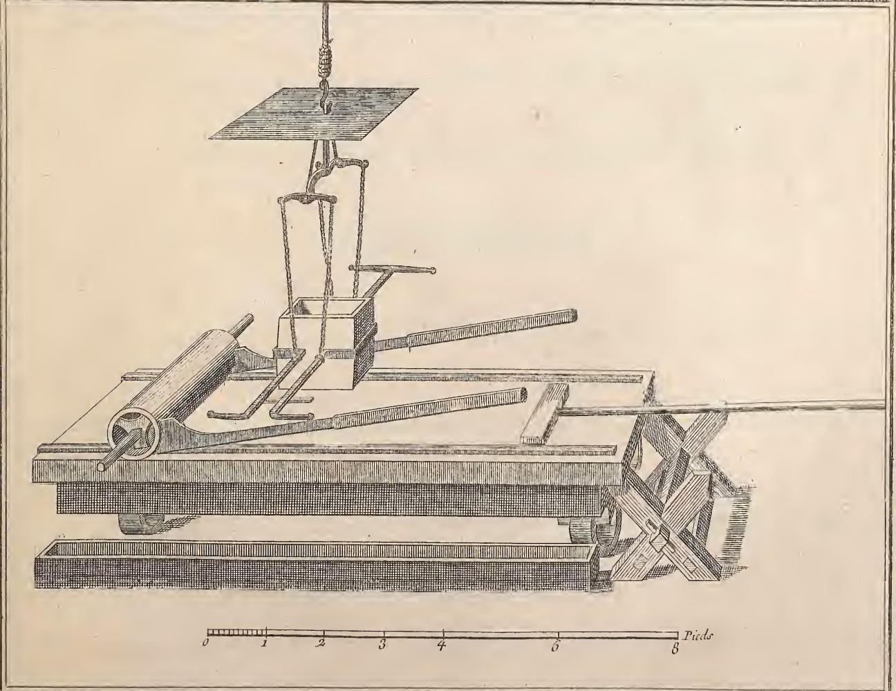
Glaces, l'opération de Verser et de Rouler.
