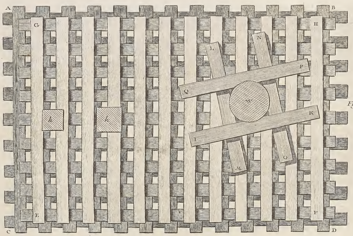
Forges, Section, Coupe Transversalle de la Forge à deux Feux et Plan de la Fondation de l'Ordon.
