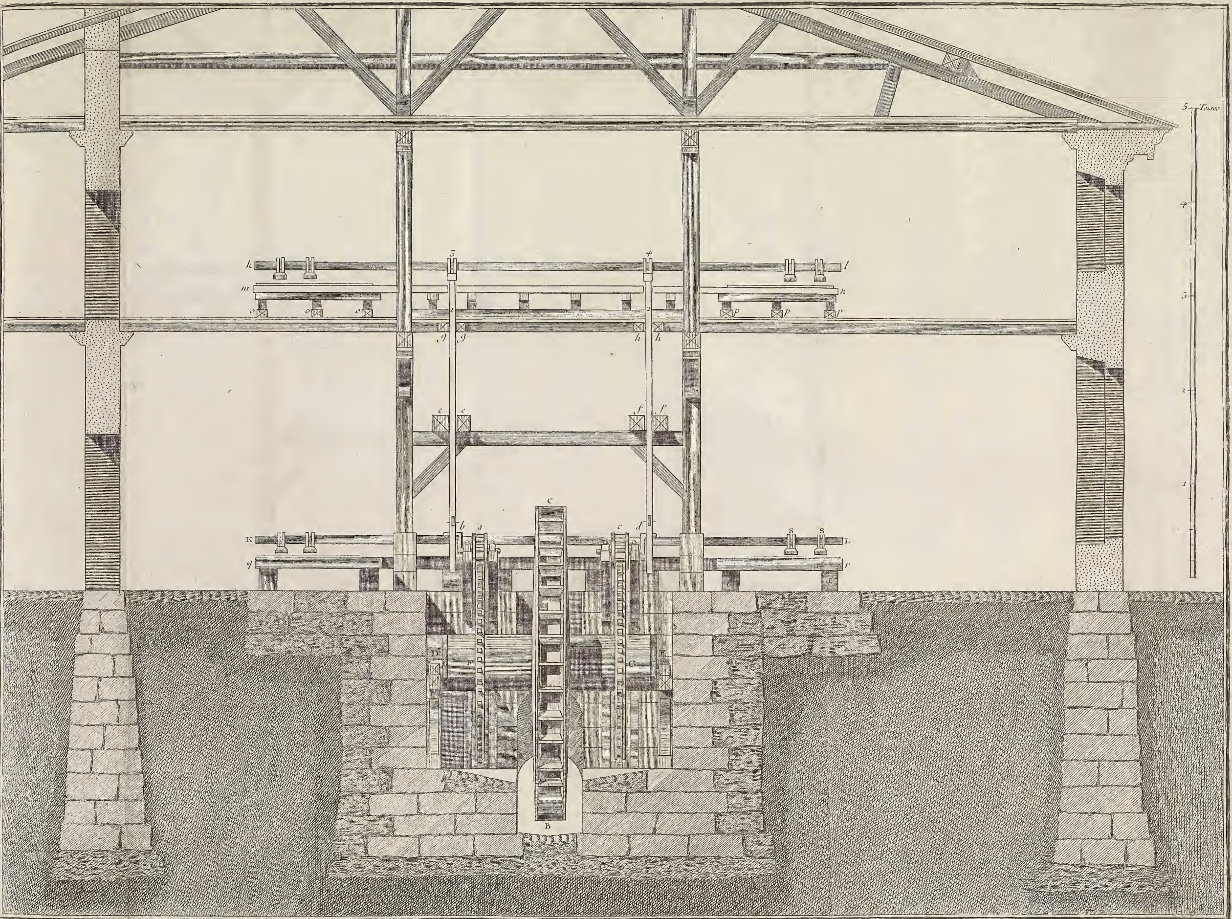
Glaces, coupe et Elevation de la Machine à polir les Glaces, prise parallèlement à l'Arbre de la Grande Roue.
