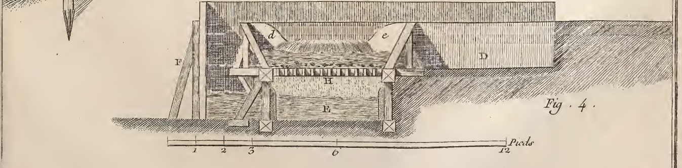
Forges, 1 re Section, Lavoir de Robert.
