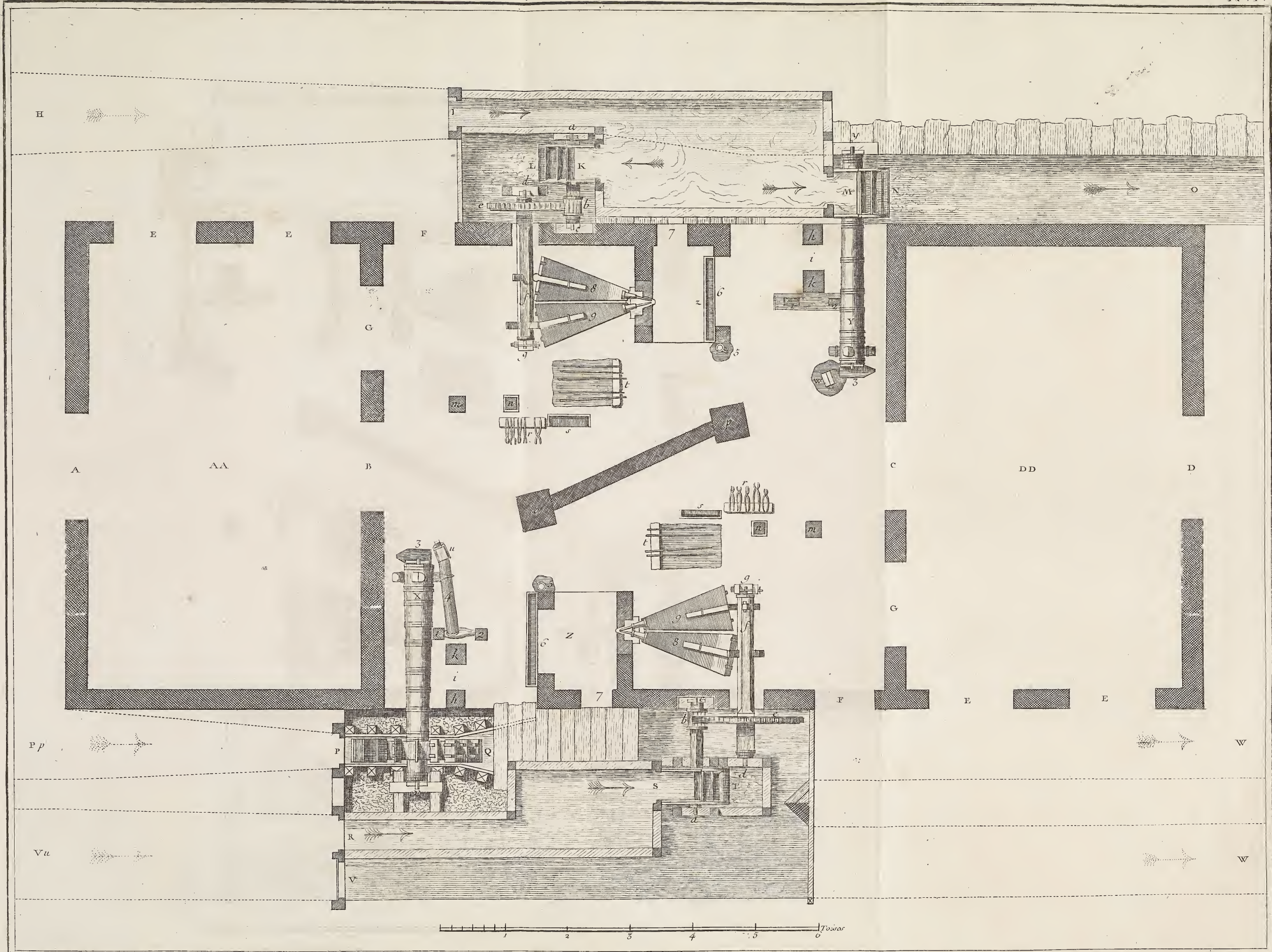
Forges, 4 e Section, Plan Général d'une Forge à deux Feux.
