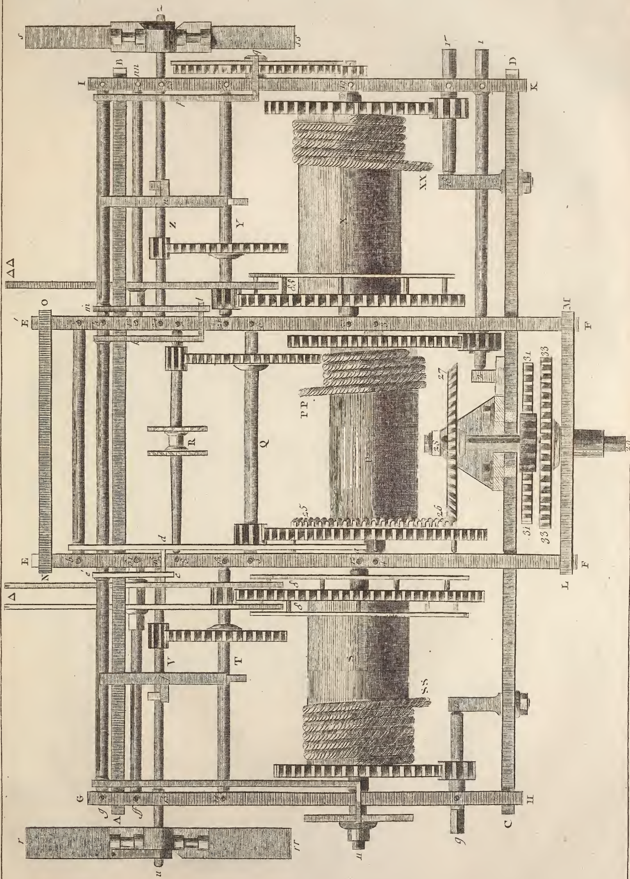
Horlogerie, plan de l'Horloge Horizontale
