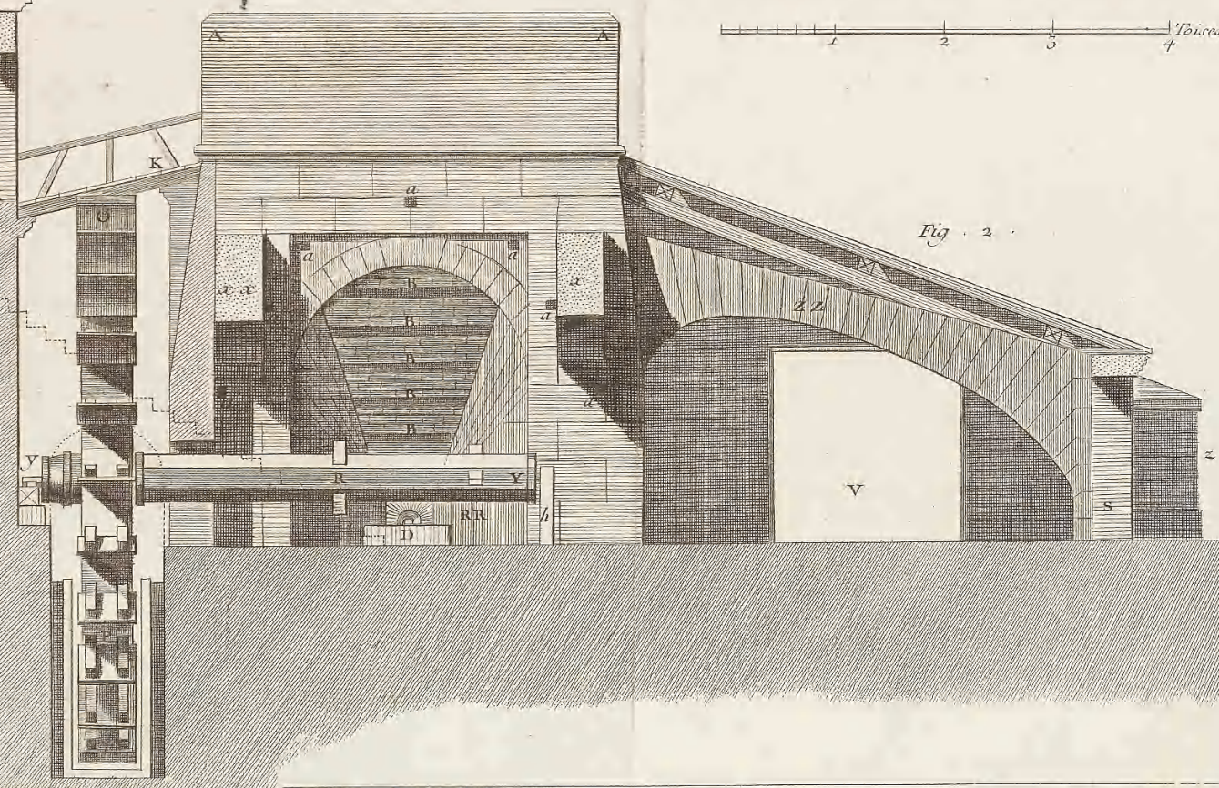
Forges, 2e Section, Fourneau à Fer, Elevations et Coupes d'un Fourneau.
