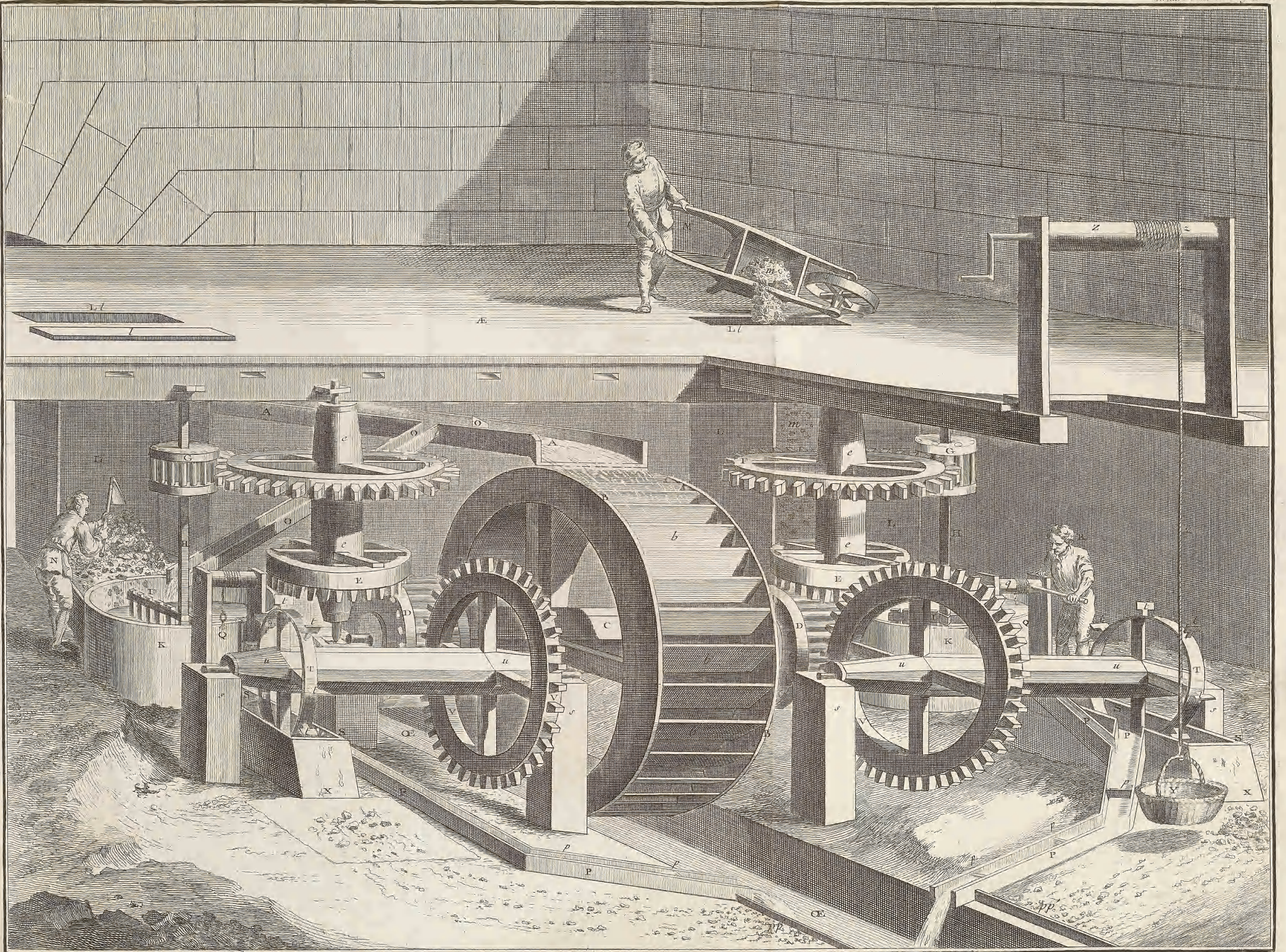
Grosses Forges, Lavage de la Mine, Vue perspective d'un Patouillet
