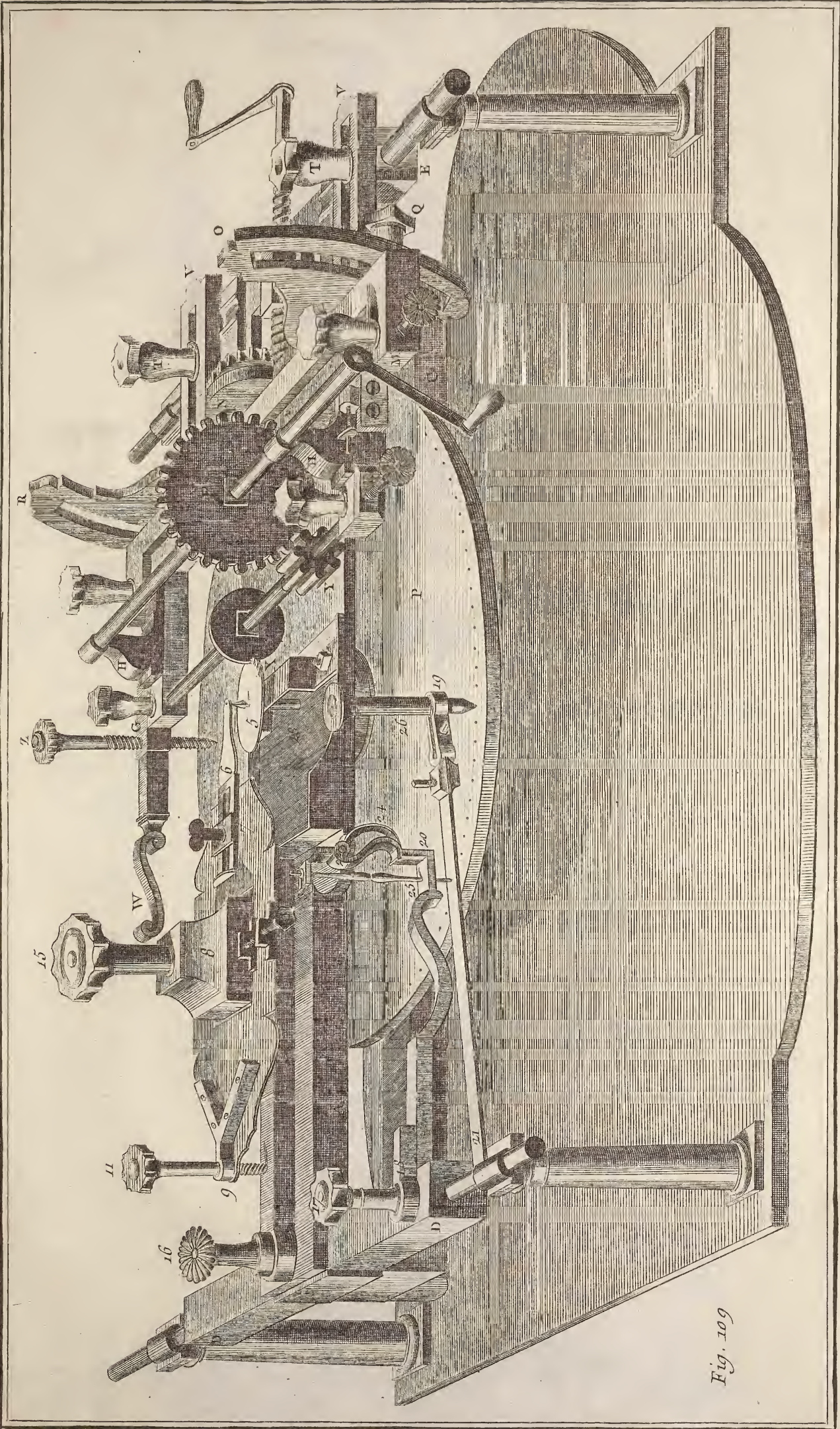
Horlogerie, Vue perspective de la Machine de Sullit pour fendre les Roues.
