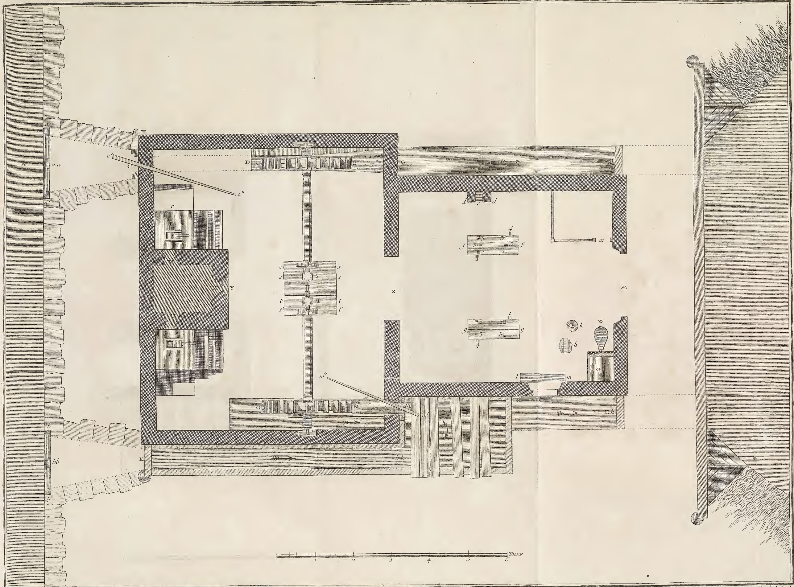
Forges, 5 e Section, Plan Général d'une Fenderie.
