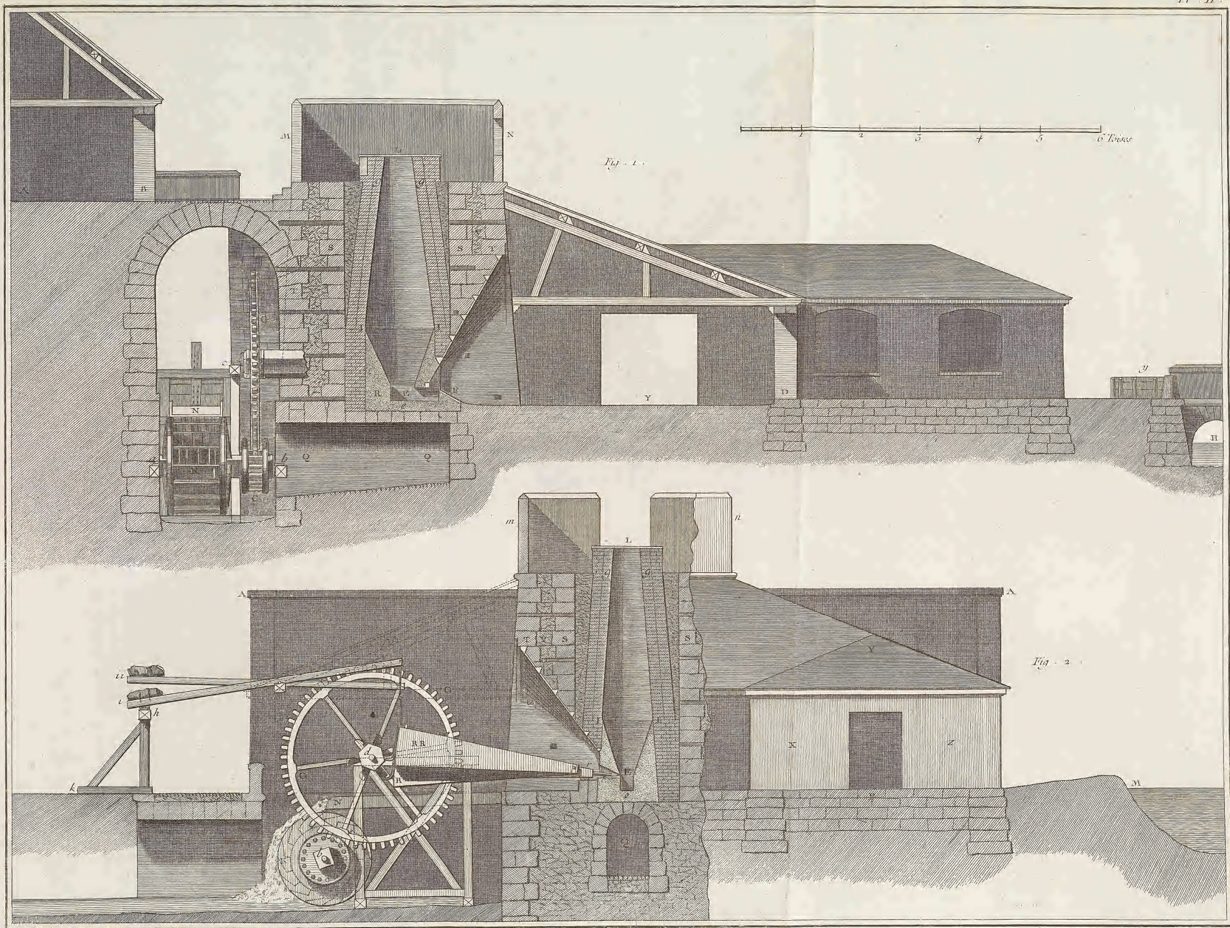
Forges, 3 e Section. Coupes d'un Fourneau en Marchandise.
