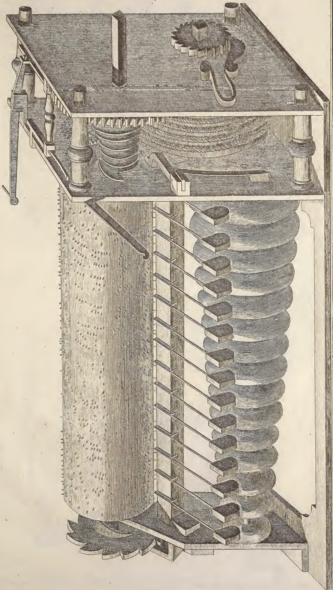
Horlogerie, un Carillon. Vue perspective d'un Carillon.
