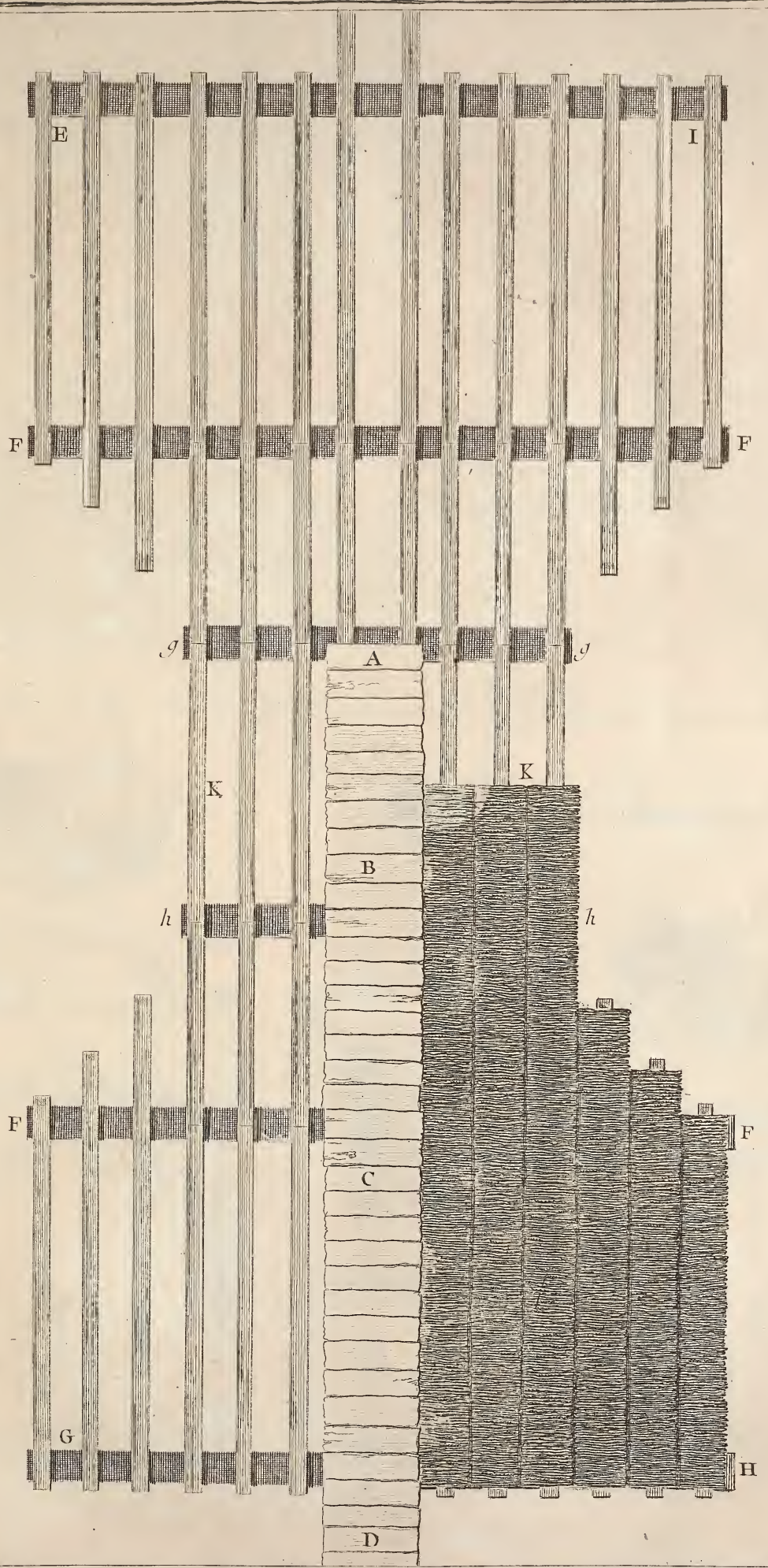
Glaces, Plan de la Roue.
