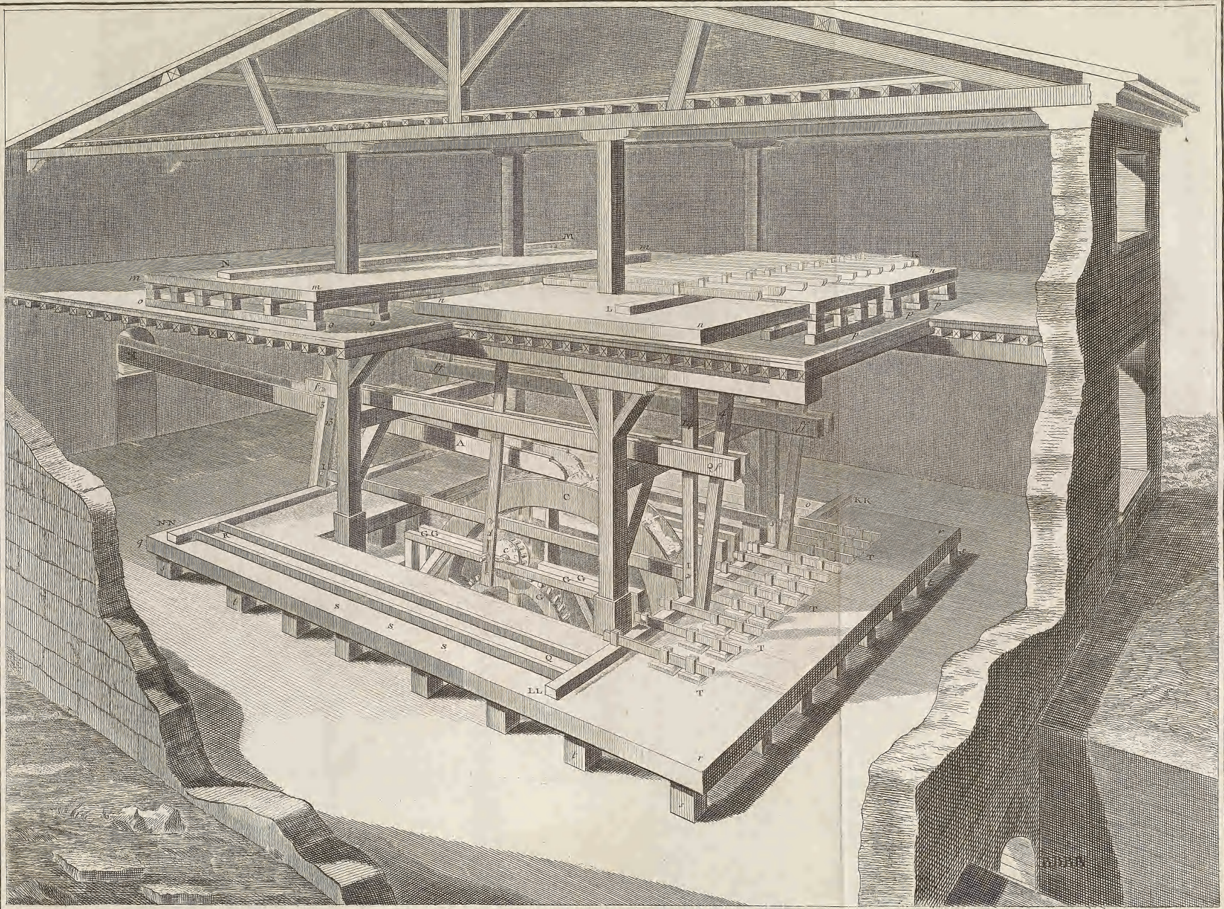
Glaces, Elévation perspective de la Machine à polir les Glaces, Etablie à St. Idelphonse.
