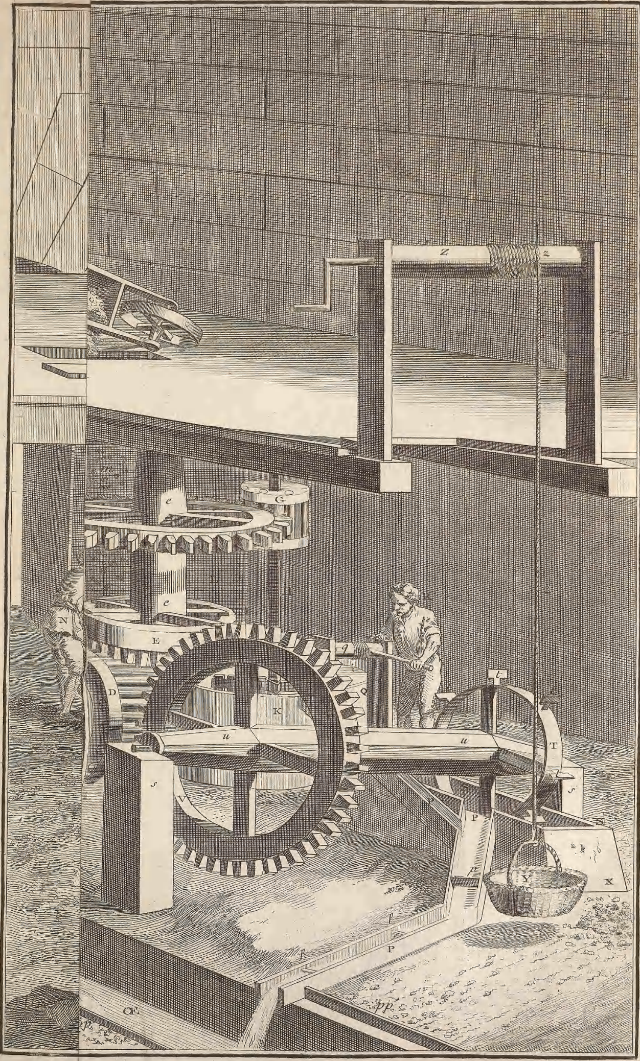
ive d'un Patouillet
