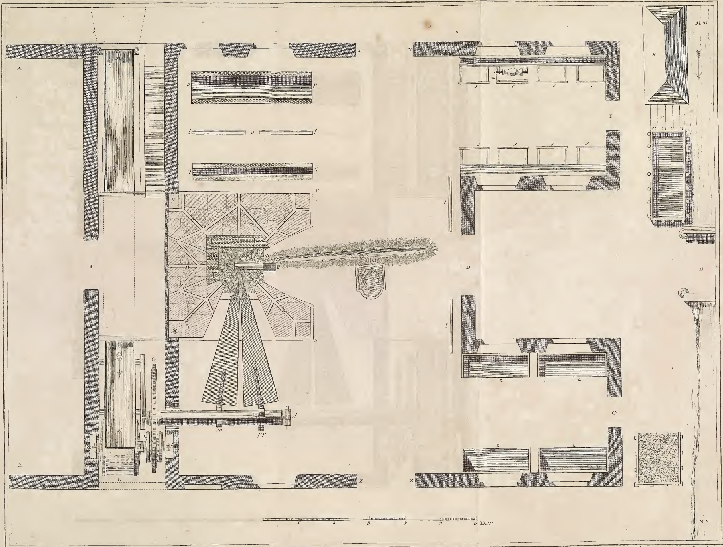
Forges, 3 e Section, Plan Général d'un Fourneau en Marchandise.
