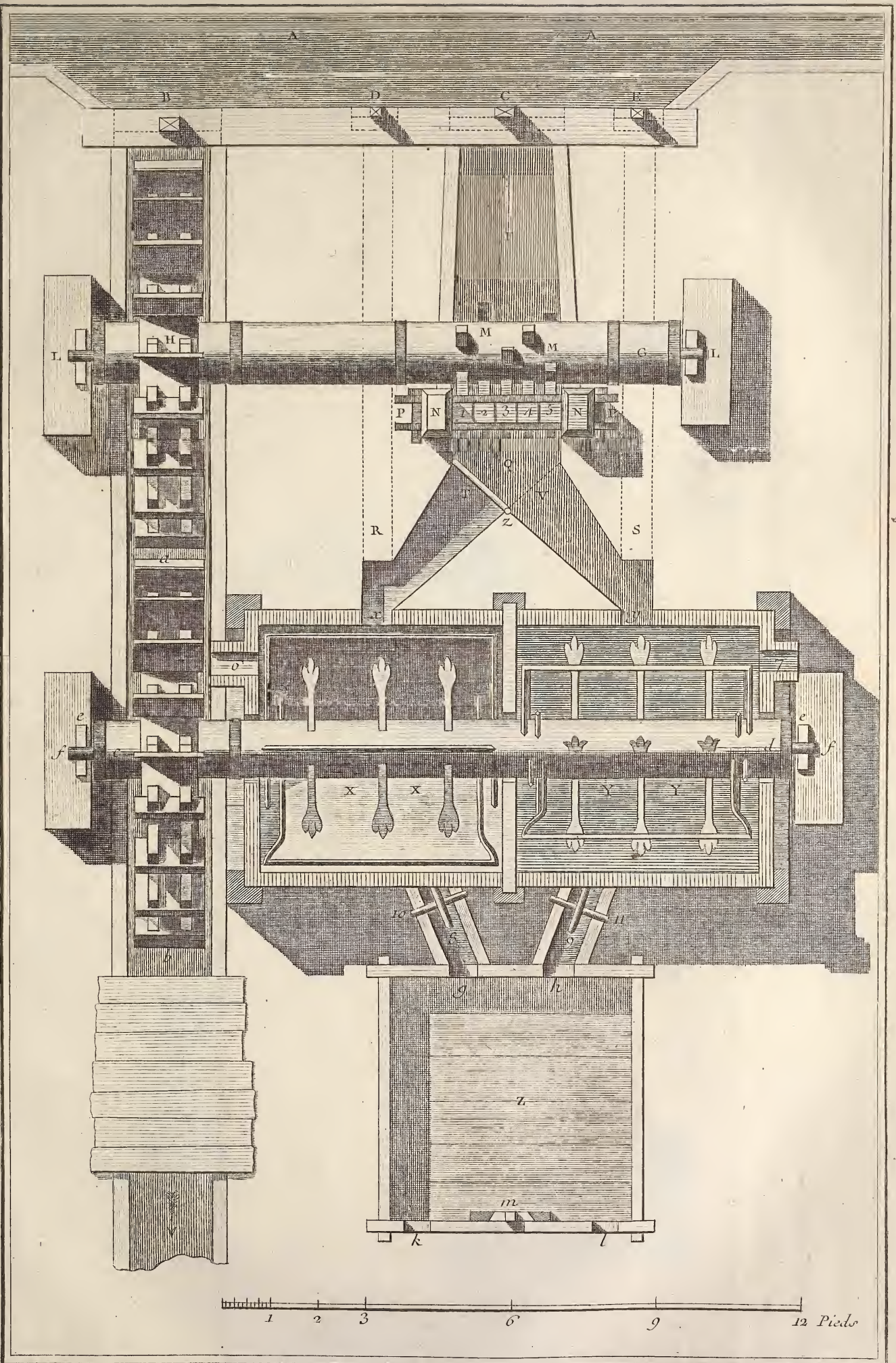
Forges, 1 re section, Bocard composé.
