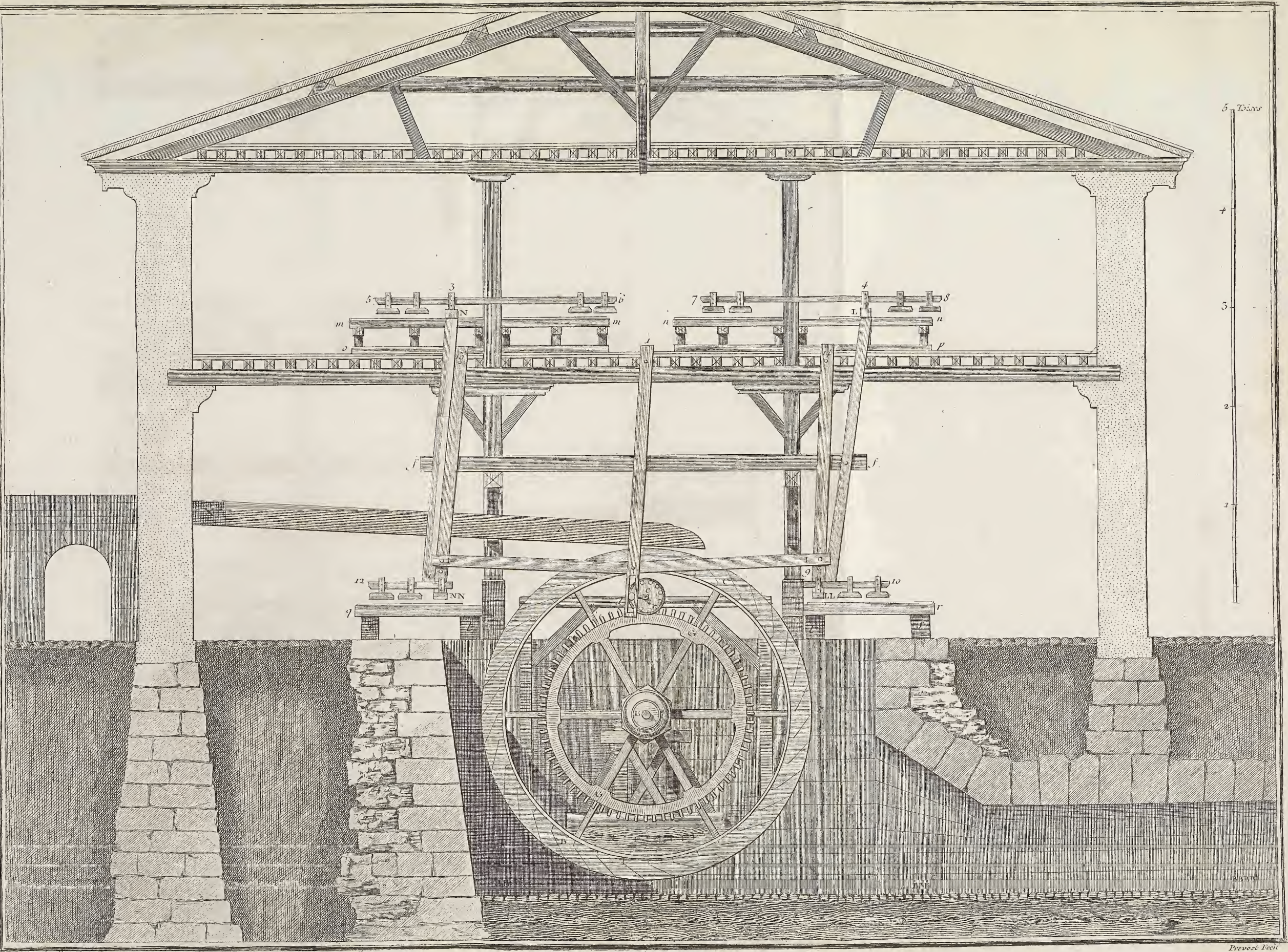
Glaces, coupe et Elévation de la Machine à polir les Glaces prise selon la longueur du Courssier.
