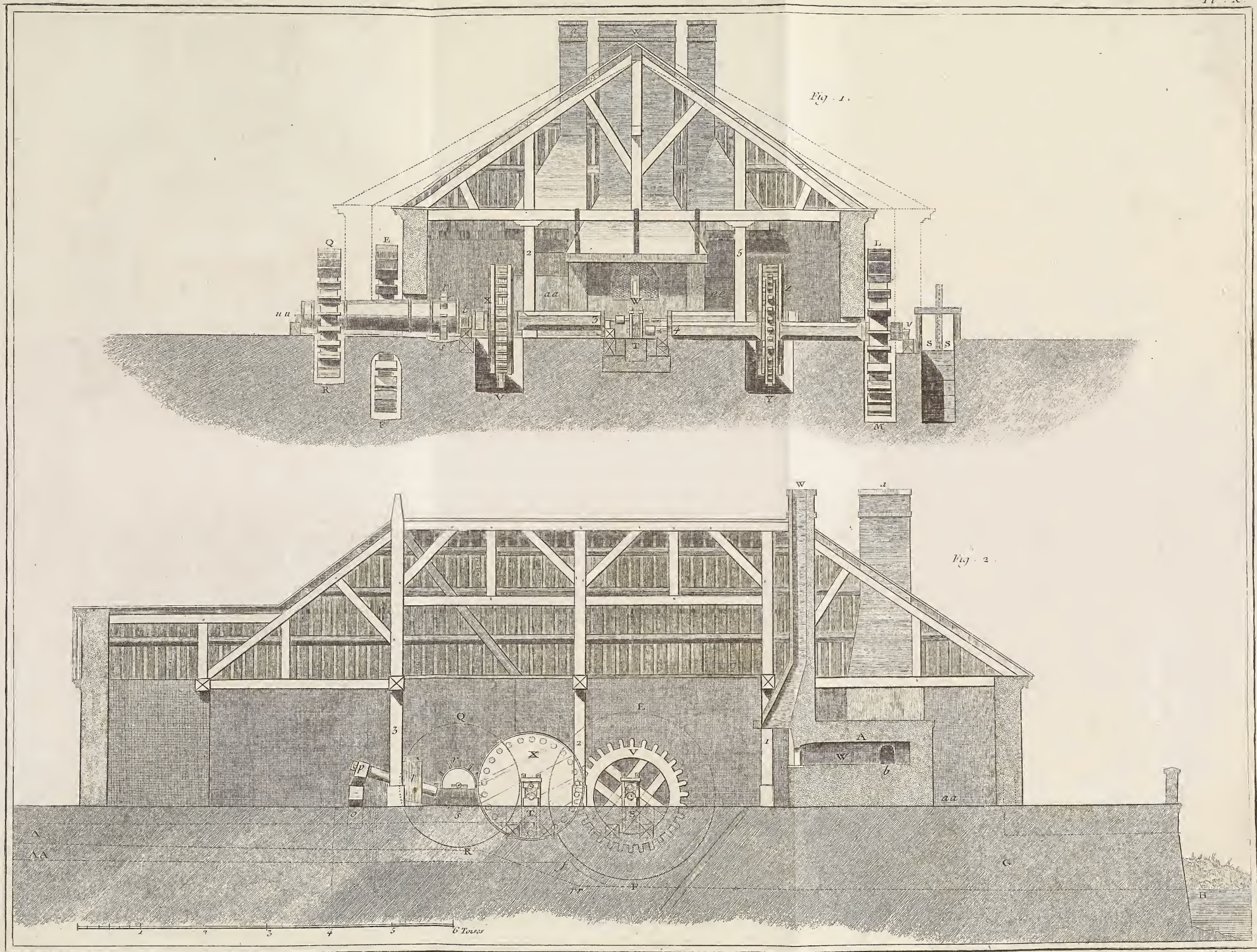
Forges, 5 e Section: Fenderie, Coupes de la Fenderie à double Harnois.
