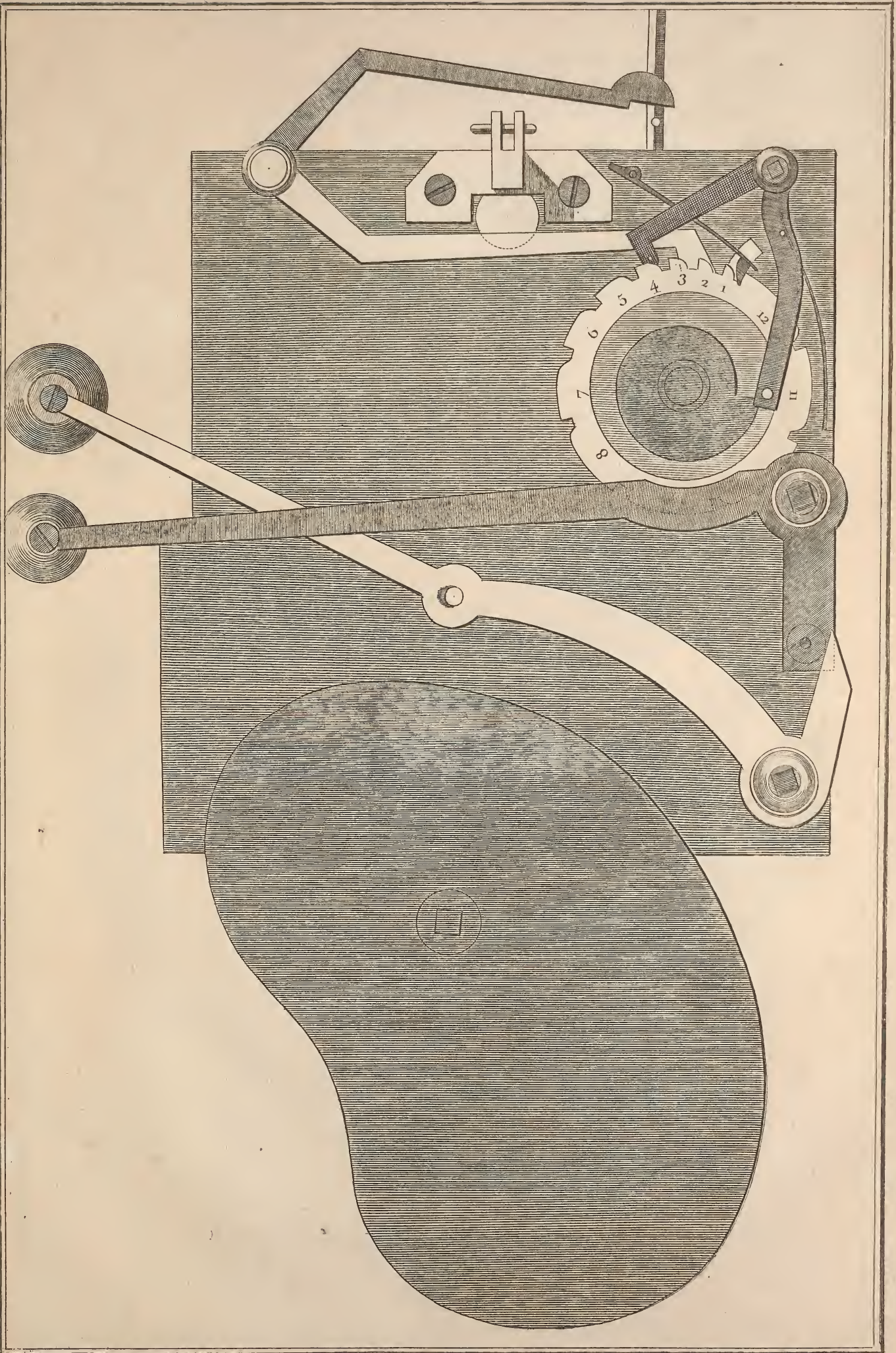
Horlogerie Pendule d'Equation de le Bon.
