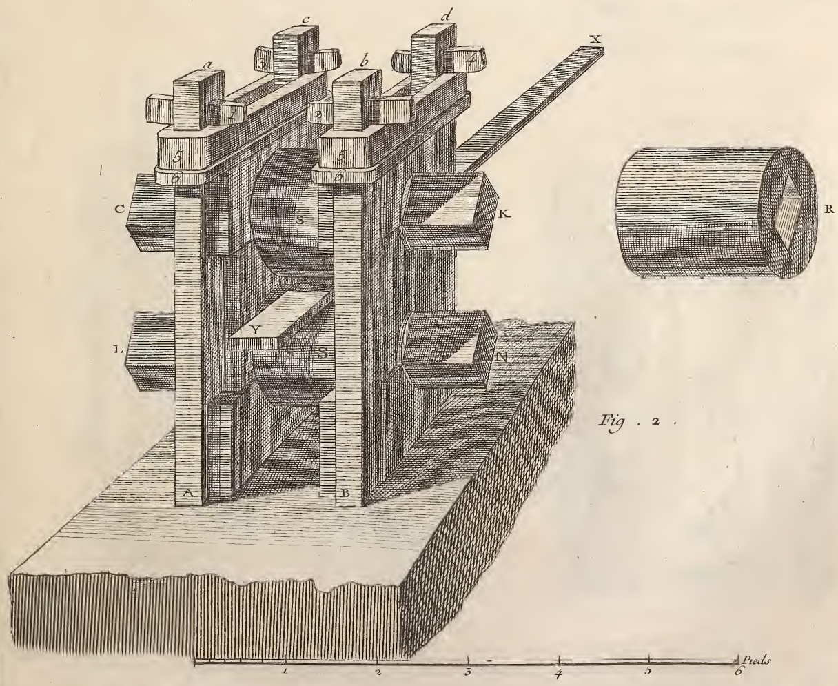
Forges, 5 Section, Fenderie, Développemens des Espatars.
