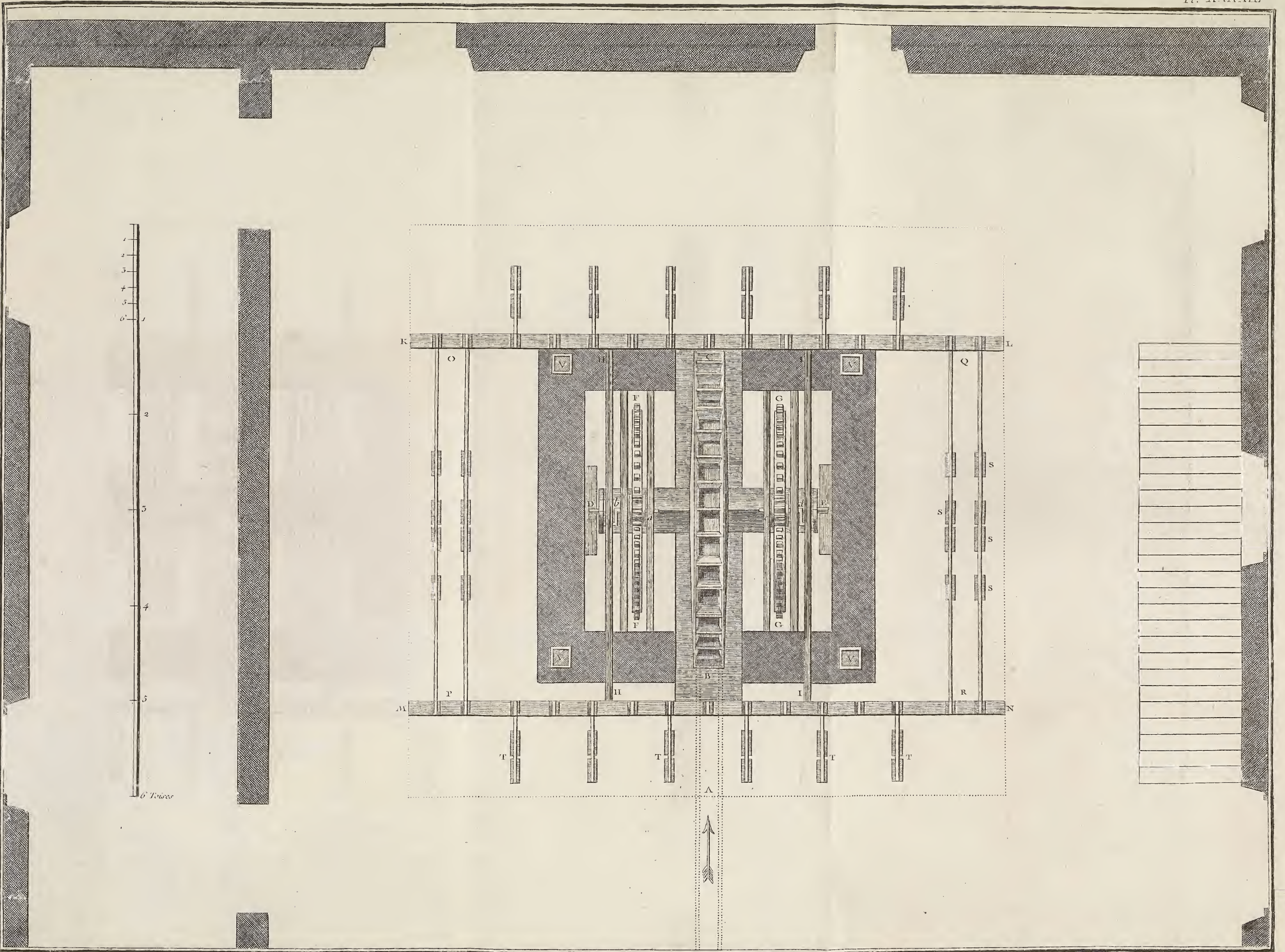
Glaces, Plan du Rez de Chaussée de la Machine à polir les Glaces, Etablie à S t Idelfonse.
