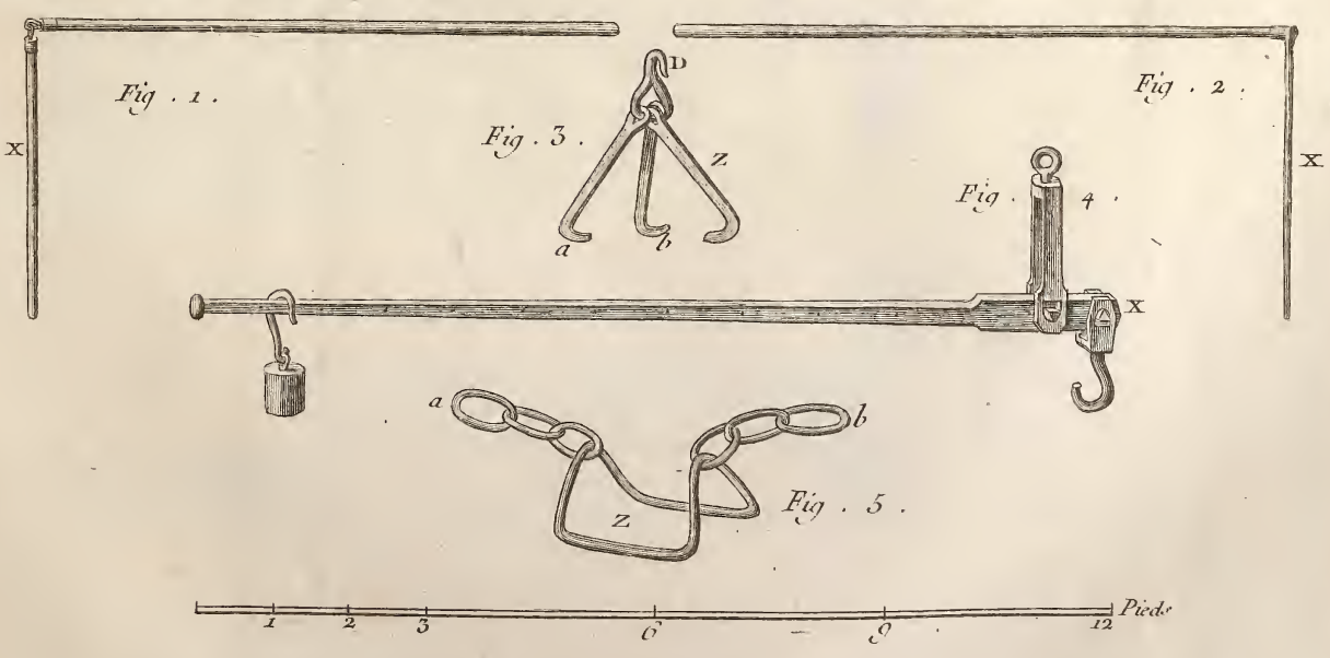
Forges ; 2 e . Section, Fourneau à Fer, Sonder et Peser.
