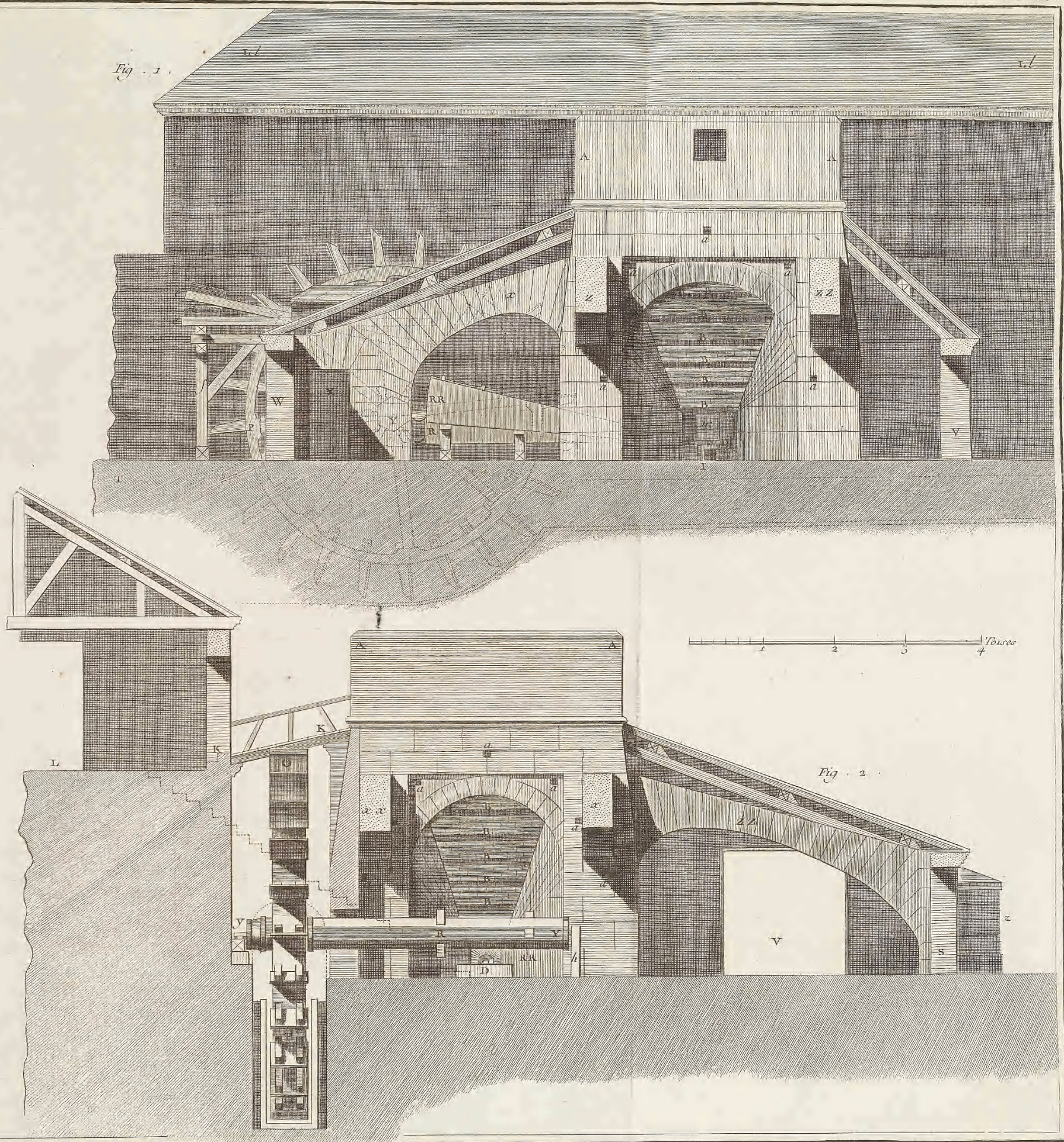
Forges, 2e Section, Fourneau à Fer, Elevations et Coupes d'un Fourneau.
