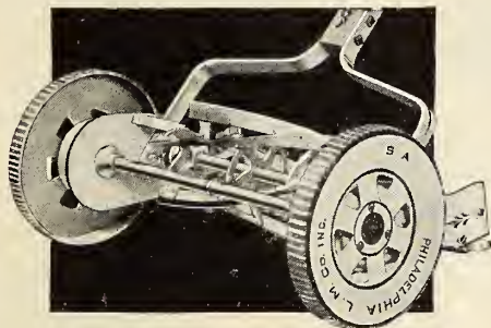
Philadelphia Style S-A Mower
