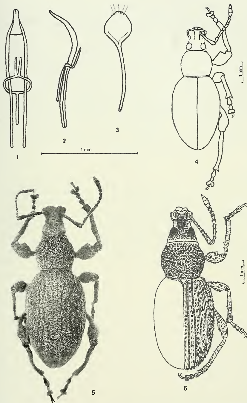
FIGG. 1-6. - 1-5: Otiorhynchus (Melasemmus?) lepidus sp. n. 1: edeago in visione dorsale; 2: edeago in visione laterale; 3: spiculum ventrale; 4: ♂, habitus, schematico; 5: habitus. - 6: Otiorhynchus relicinus habitus, schematico, da Arnoldi, 1975.
