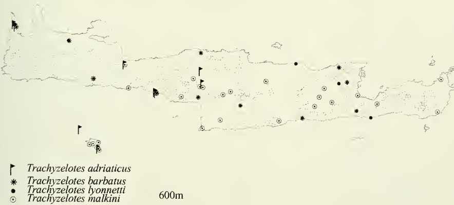
FIG. 117 Trachyzelotes adriaticus , T. barbatus , T. lyonnetti , T. malkini , distribution on Crete.
