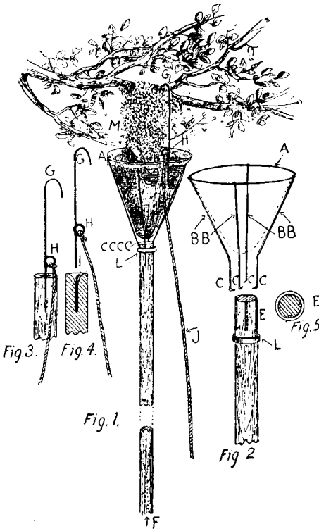
Роевня для снятия роевъ съ высокихъ деревьевъ.
