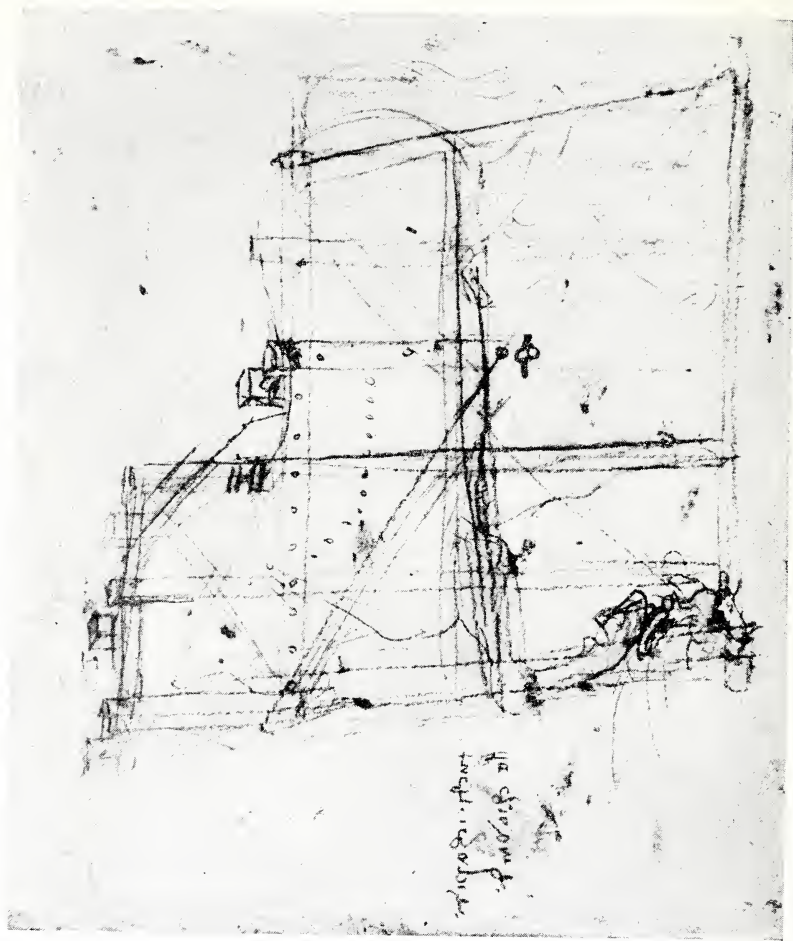
LEONARDO - SCHIZZI PER LA FUSIONE (Windsor, Biblioteca reale ), E PER L'ARMATURA DEL CAVALLO (Milano, Biblioteca Ambrosiana , « Cod. Atlantico », fol. 216 a).
