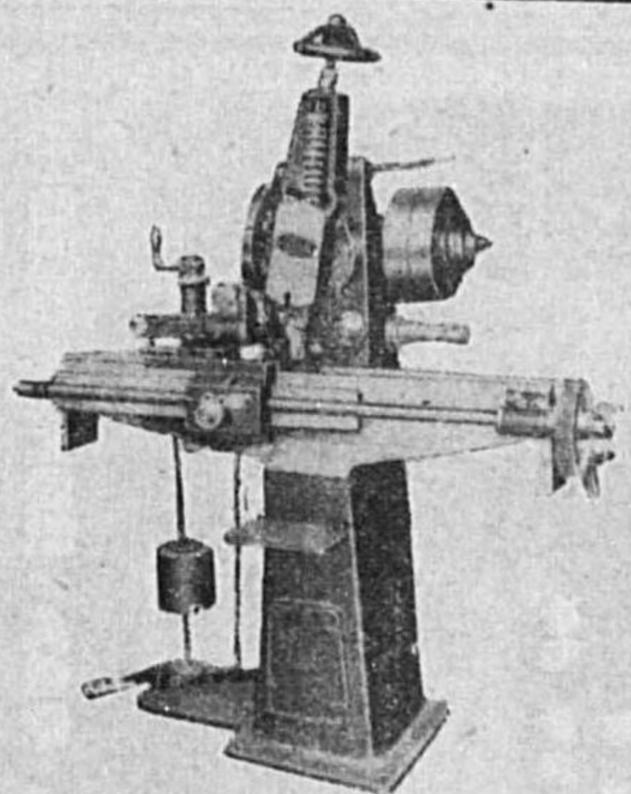
鑄製作機
