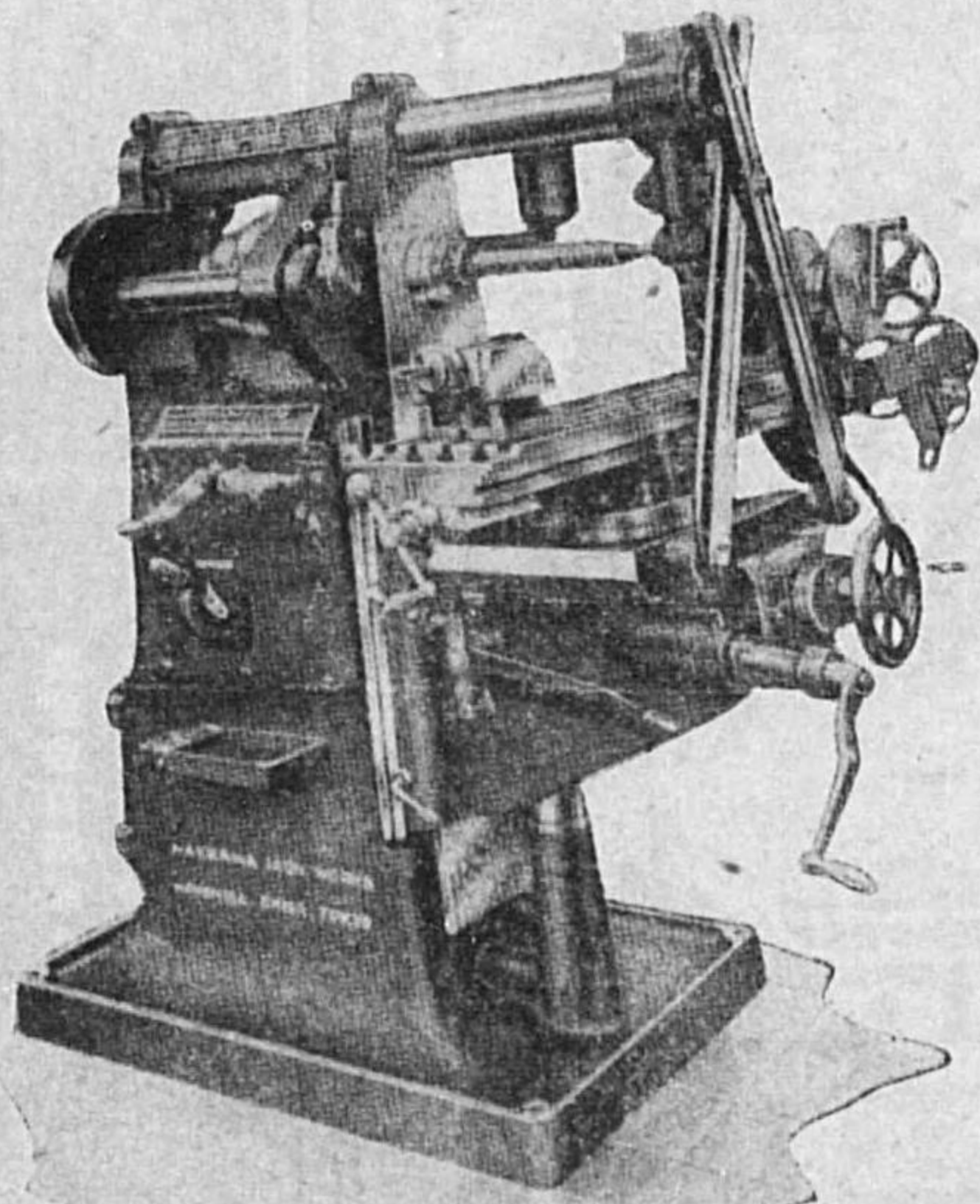
No. 2 ユニバーサルミーリングマシン
