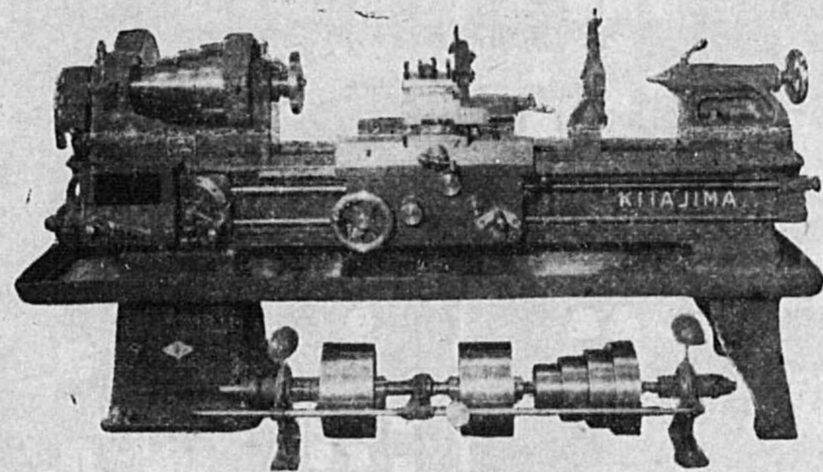
北島 400×2000 耗 B 型 米式旋盤
