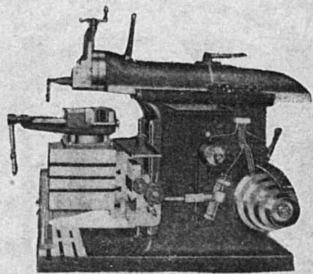
(二〇吋成形機)
