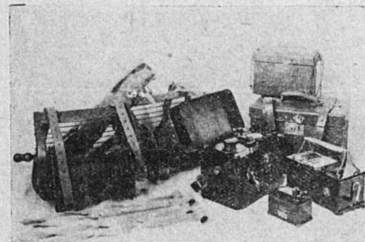
地質試験器
